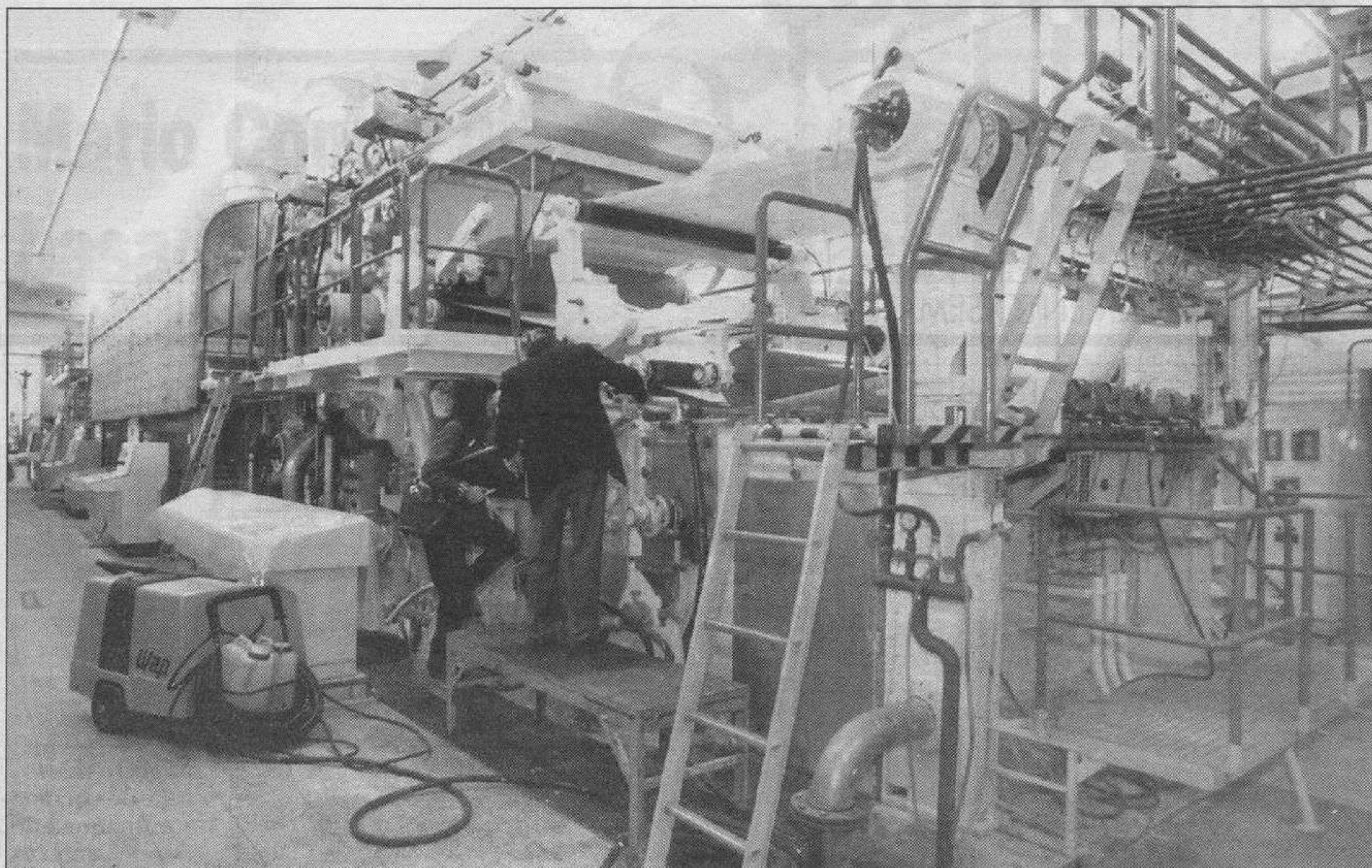
La máquina de papel consta de seis secciones. En 1992 sufrió una gran modificación tecnológica. A la drcha., el director de la Fábrica, Pedro Guzmán.
