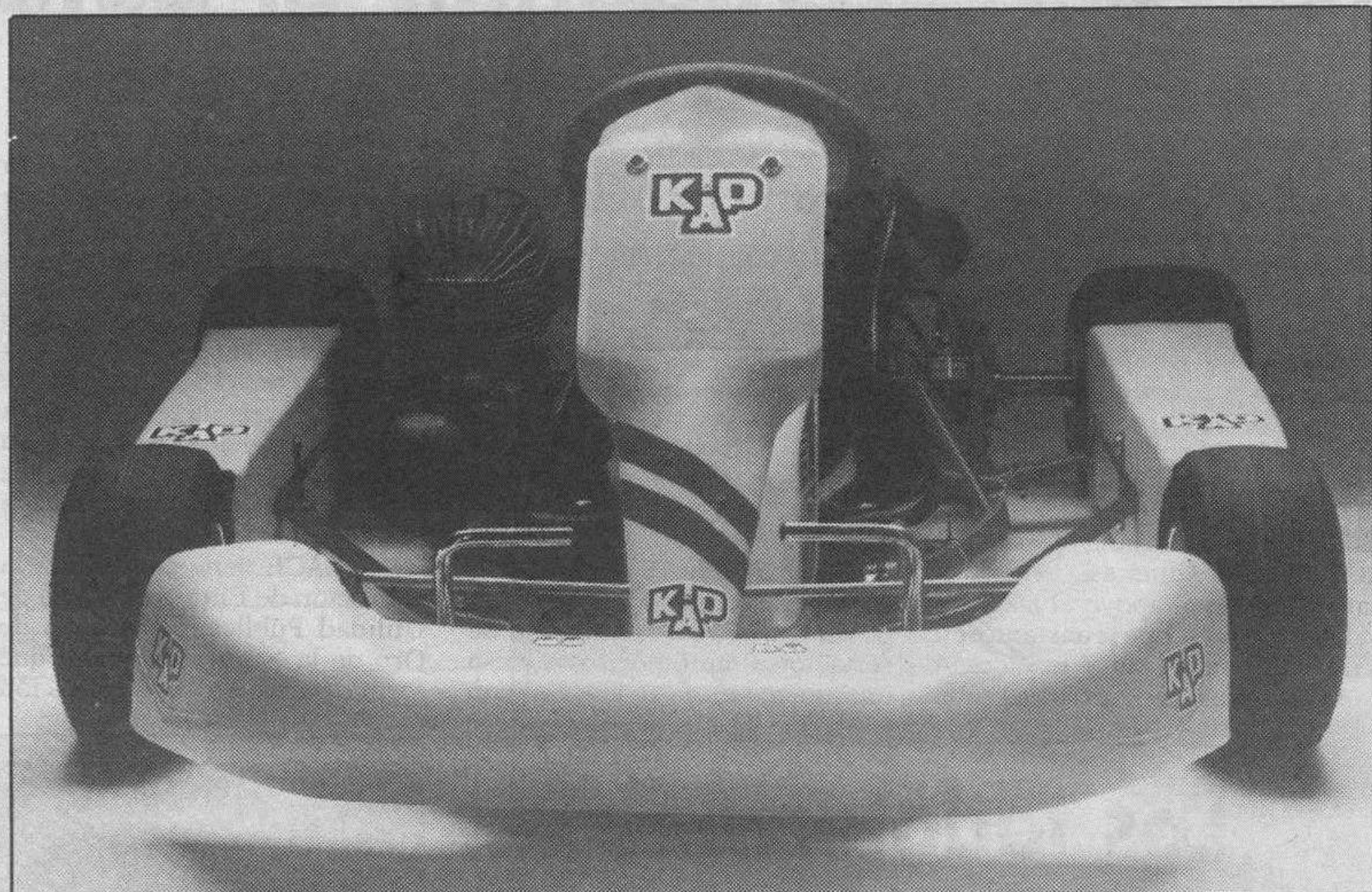
La caída de las ruedas delanteras asegura la mejor adherencia al suelo
