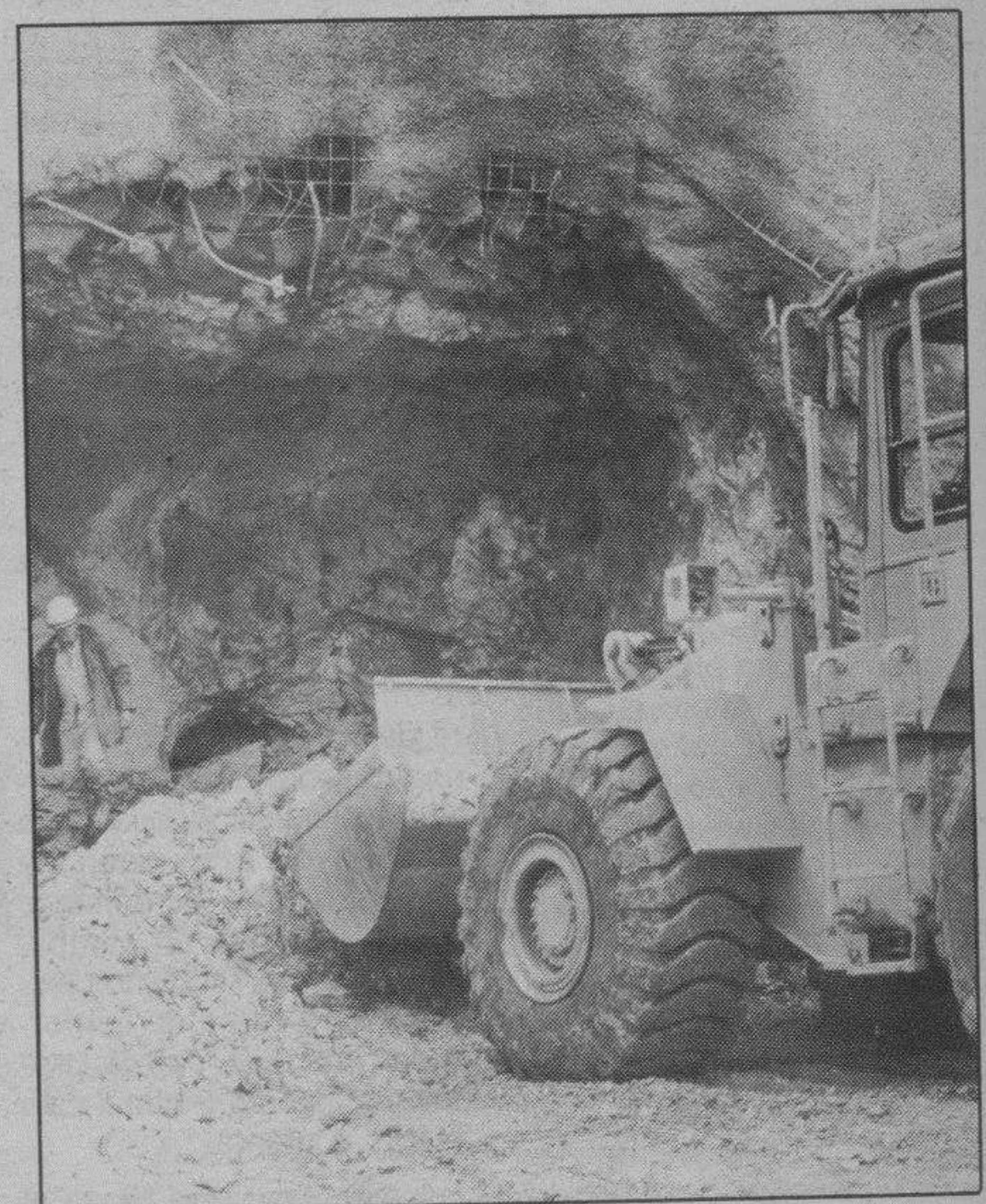
Una gran polvareda de humo y piedras, junto con un gran estruendo, se produjo con la explosión, tras lo cual y, después de esperar hasta que quedase bien visible la zona, se procedió al desescombre de lo derruido.
