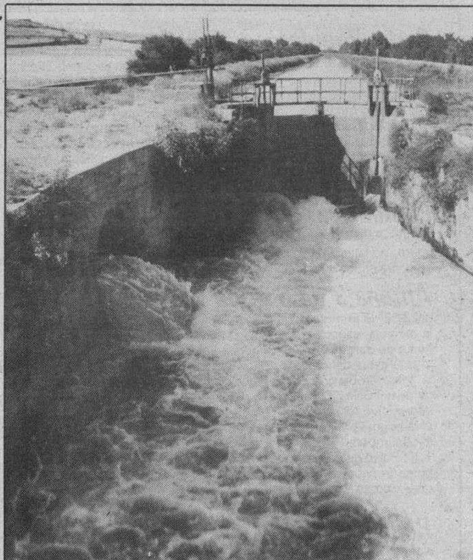
Vistas del Canal de Castilla a su paso por Melgar de Fernamental: esclusa y puente-acueducto sobre el río Abánades, conocido como «Puente del Rey».
