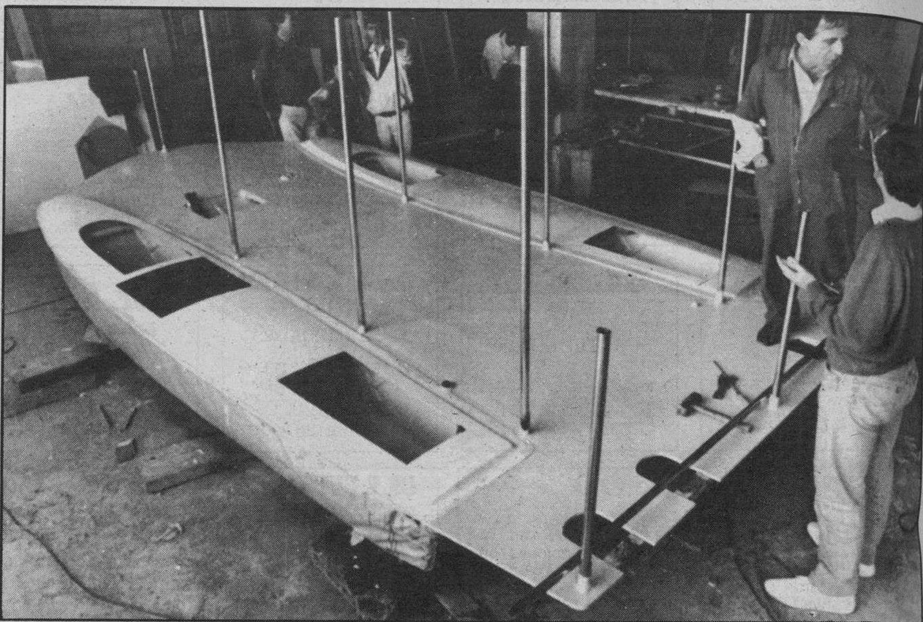
Prototipo de barco, capaz de recoger del mar separándolo, el agua de toda clase de combustibles, gasoil, petróleo, crudos, con una capacidad de recuperación de 33 toneladas por hora. Sobre el barco José San Martín y al fondo Angel Perera, sus inventores. —Telefoto Efe.
