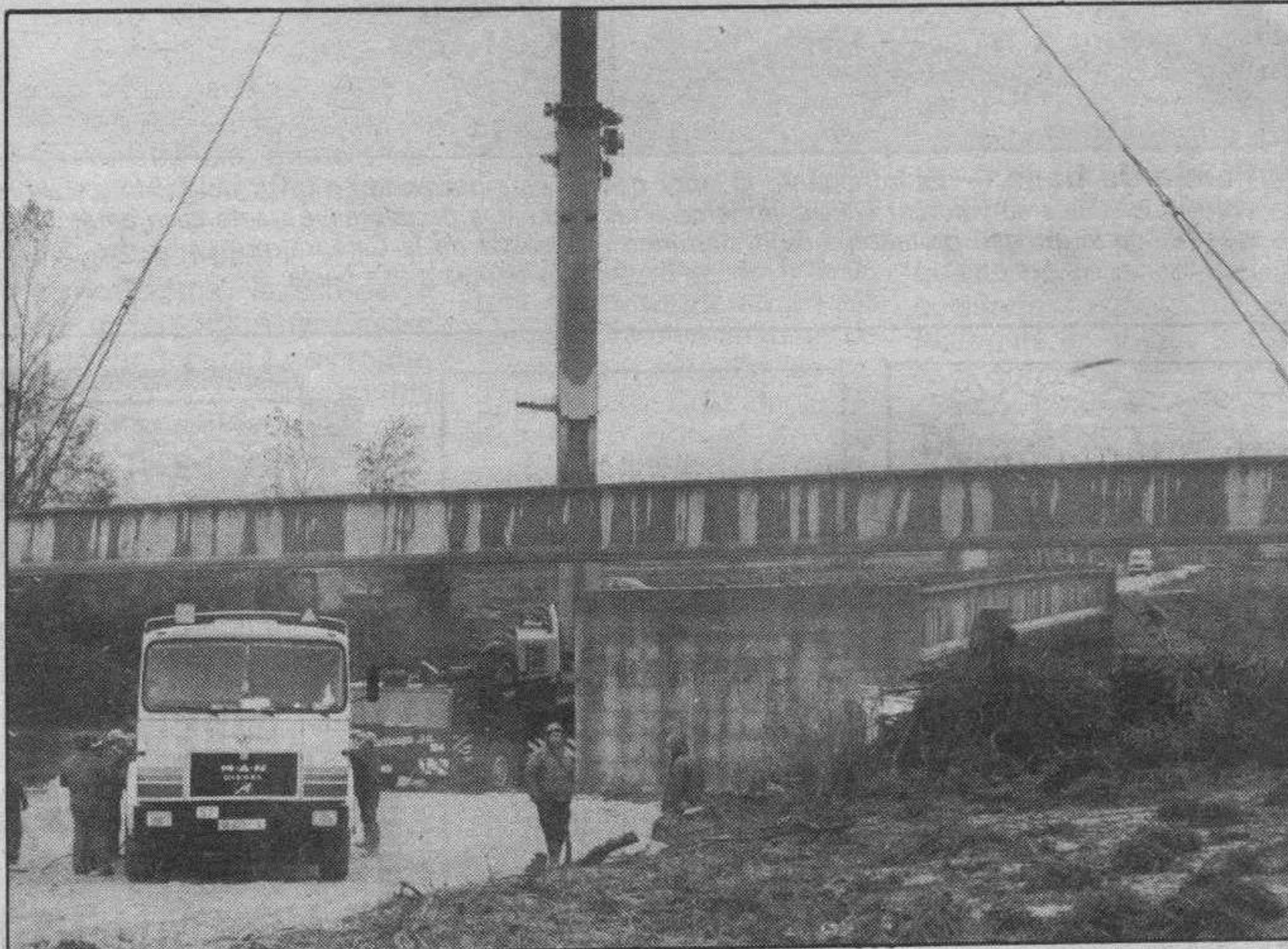
Espectacular operación sobre el Nela.— El director general de Estructuras Agrarias de la Junta de Castilla y León, José Antonio González presenció ayer en la zona de Villarcayo de la Merindad de Castilla la Vieja la espectacular operación de tendido de un puente sobre el Nela, momento que recoge la fotografía.
