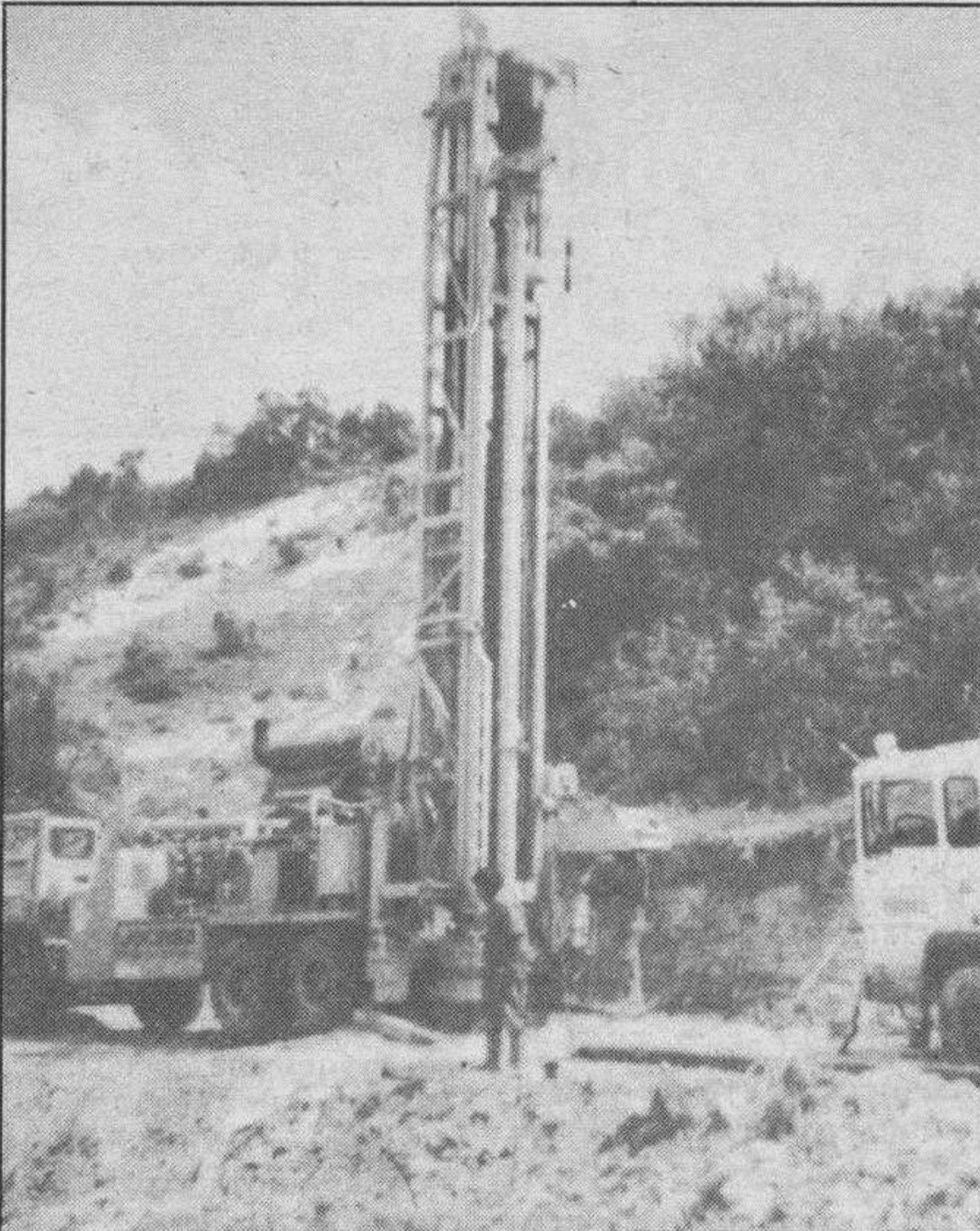
Equipo de sondeo realizando la perforación en Pedrosa Tobalina.
