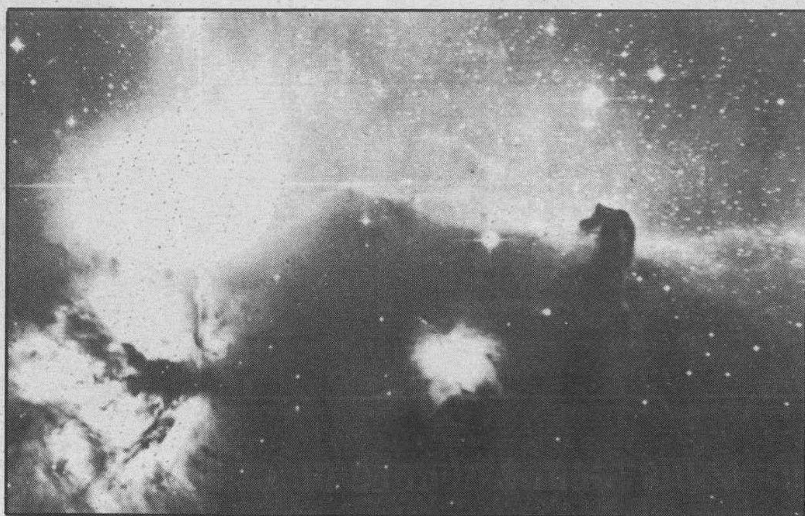
Nebulosa «Bahía Negra» en Orión, también llamada «Cabeza de Caballo».
