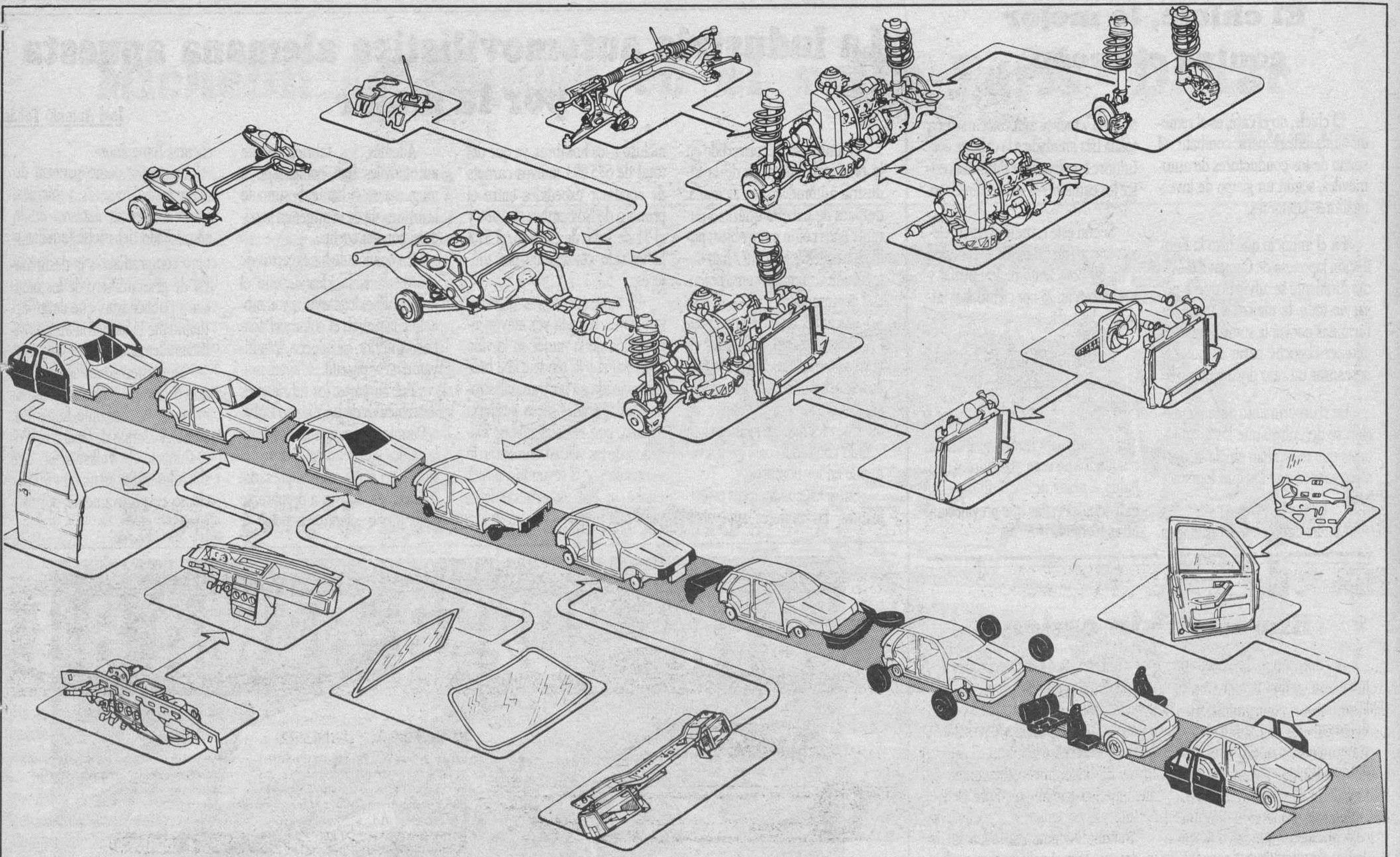
Montaje automático con grupos preensamblados fuera de línea
