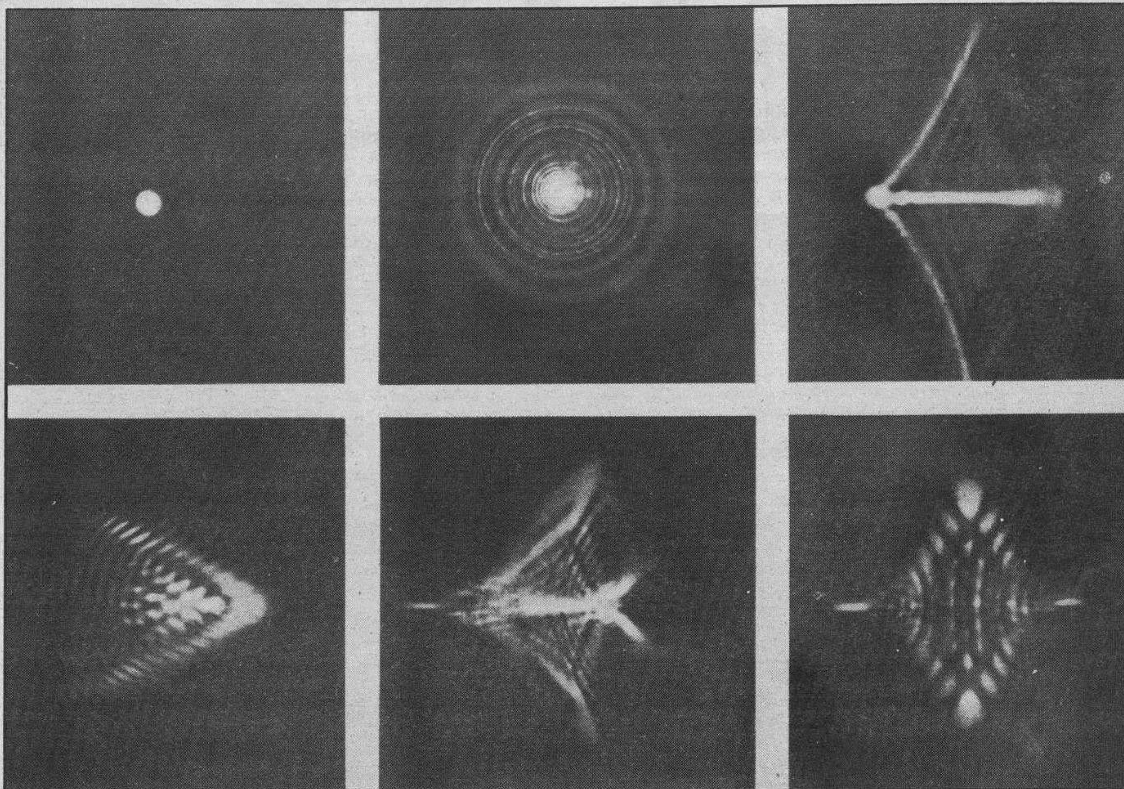
Posibles aberraciones ópticas de una estrella (punto luminoso) fotografiada a través de un objetivo sin las oportunas correcciones. Son efectos indeseables que se deben evitar en astrofotografía.
