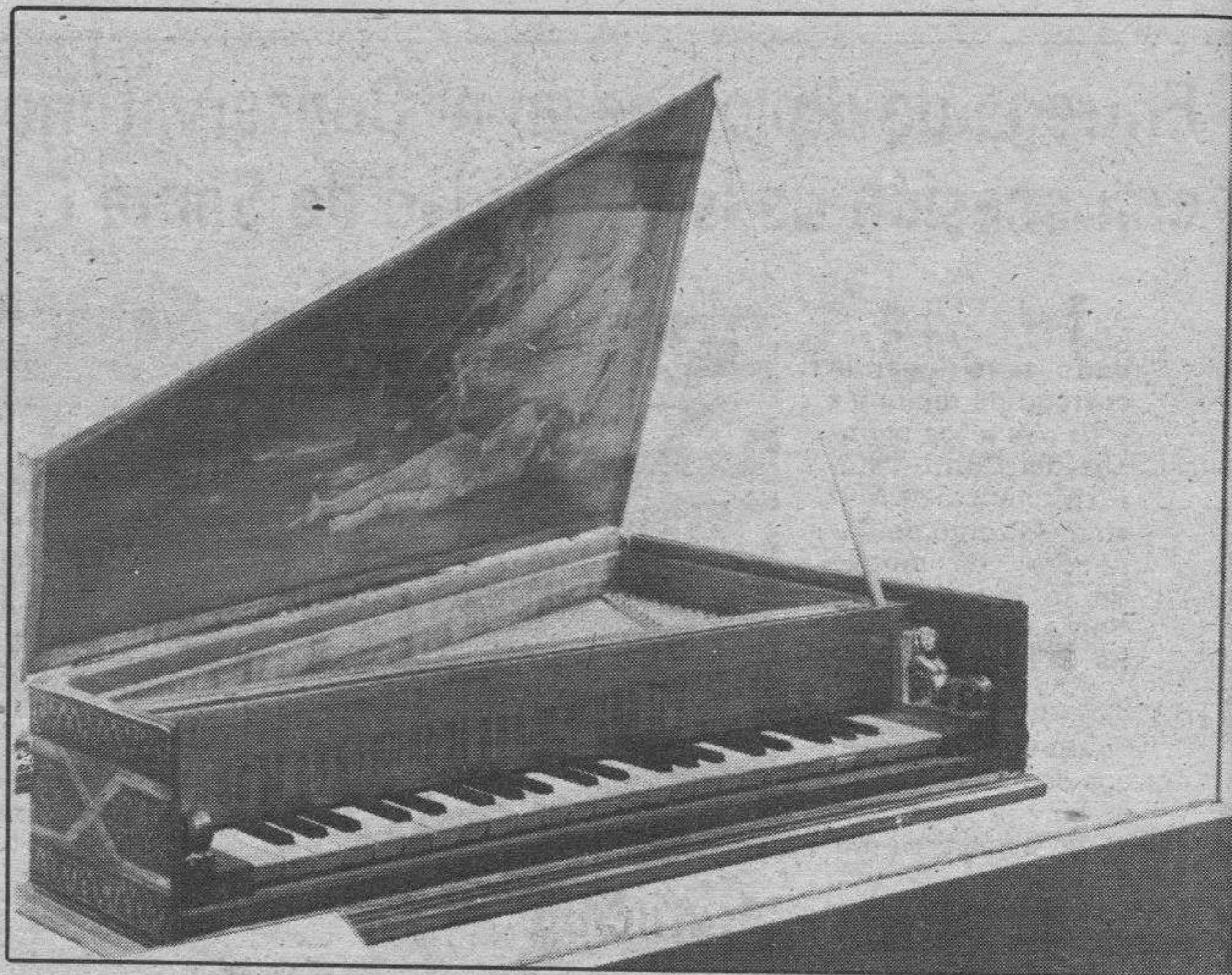
Espinet a la octava de cuatro pies. El trabajo de su construcción ha sido coordinado por Luis Joaquín Rivas Arroyo.
