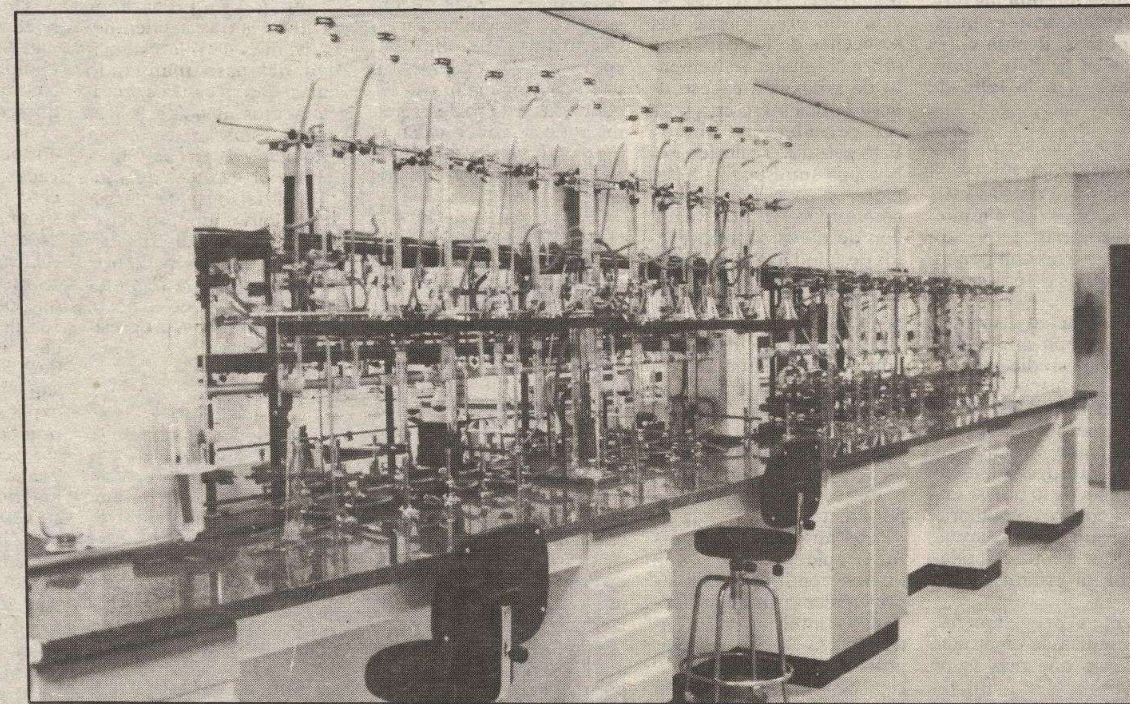
Estación Enológica de Castilla-León. Laboratorio. Equipos de análisis para la determinación del grado alcohólico, acidez volátil y sulfuroso libre y total por métodos oficiales.
