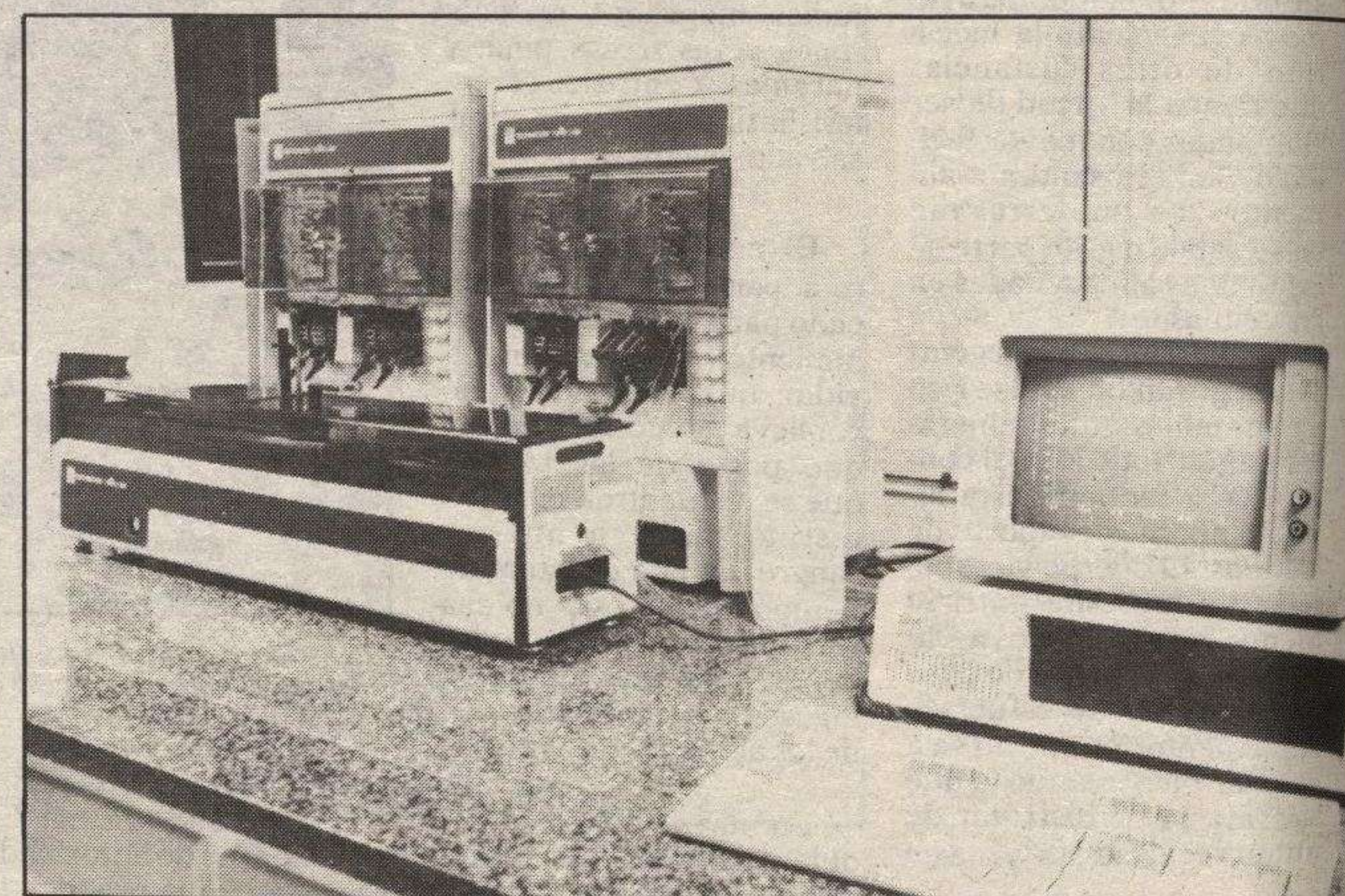
Estación Enológica de Castilla-León. Autoanalizador para 60 muestras/hora, con ordenador incorporado.
