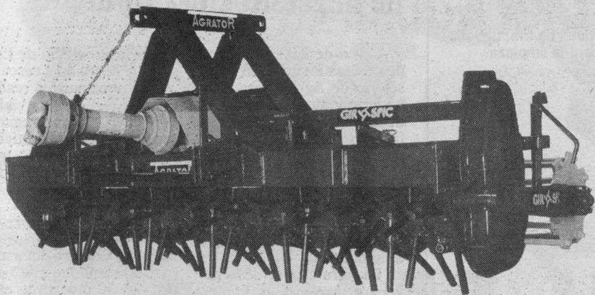
DESTERRONADORA ROTATIVA
