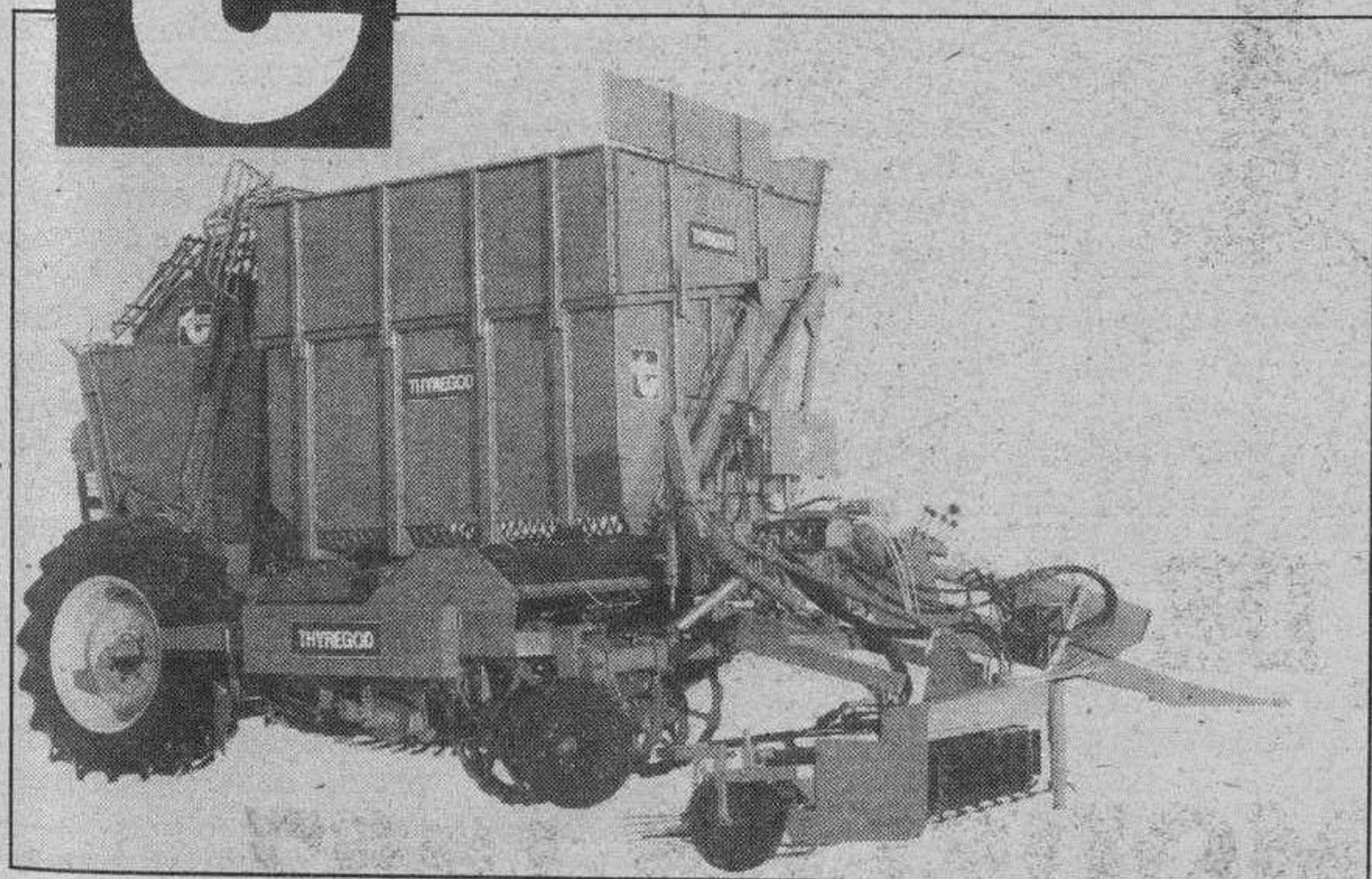
COSECHADORA REMOLACHA. TRES HILERAS
