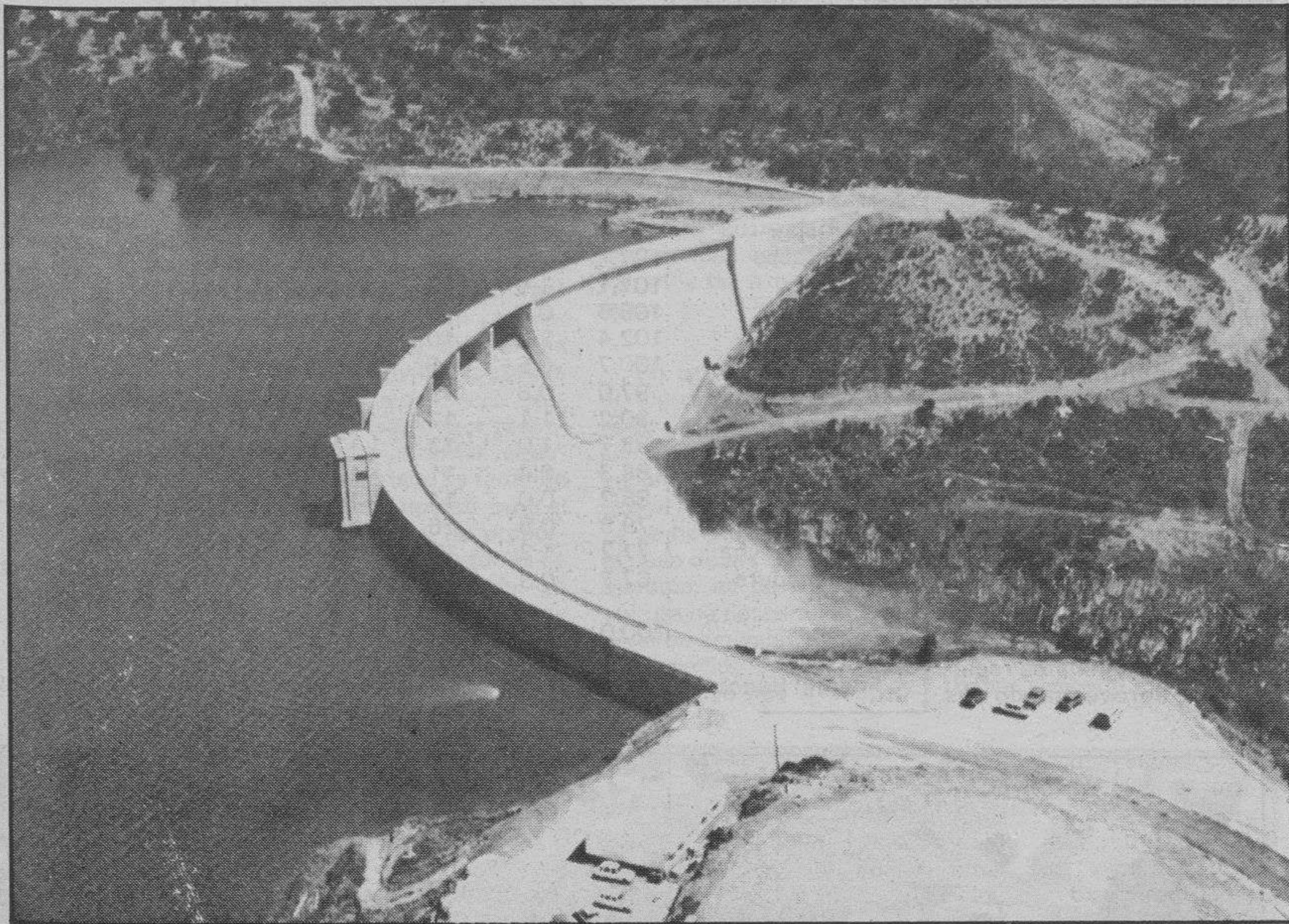
Presa del Gerbal.
