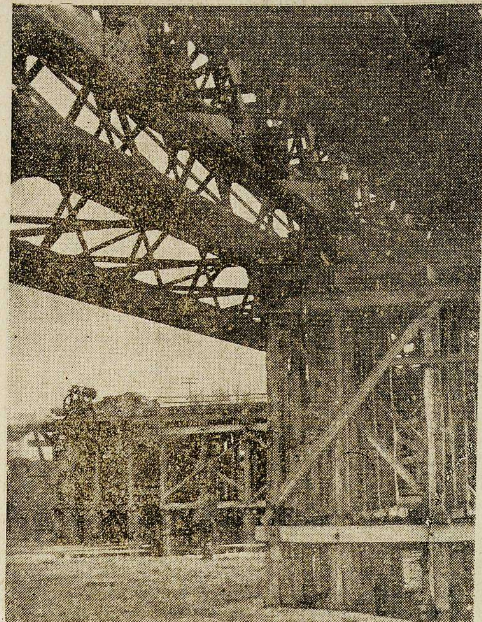
Castilletes de madera sobre los que se ha montado el nuevo puente, y los destinados a sustentar provisionalmente el viejo, al ser corrido
