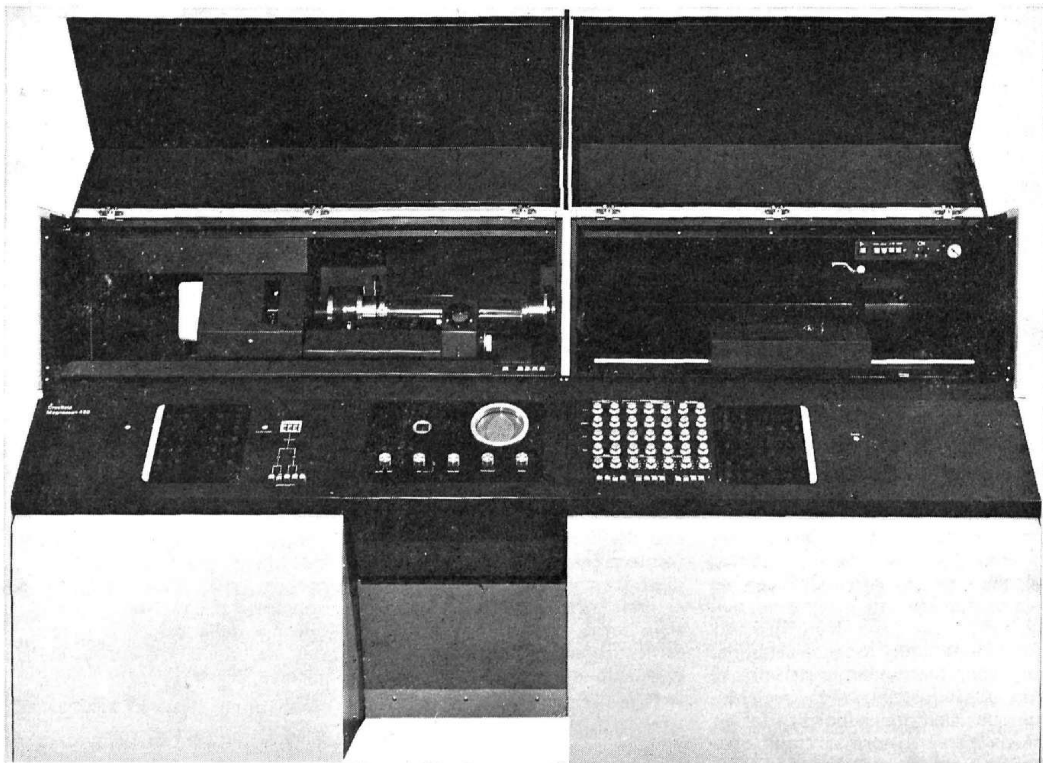
El equipo «Magnascan», analizador de color, que produce imágenes ampliadas y tramadas, con excelente calidad, detalle y rapidez.
