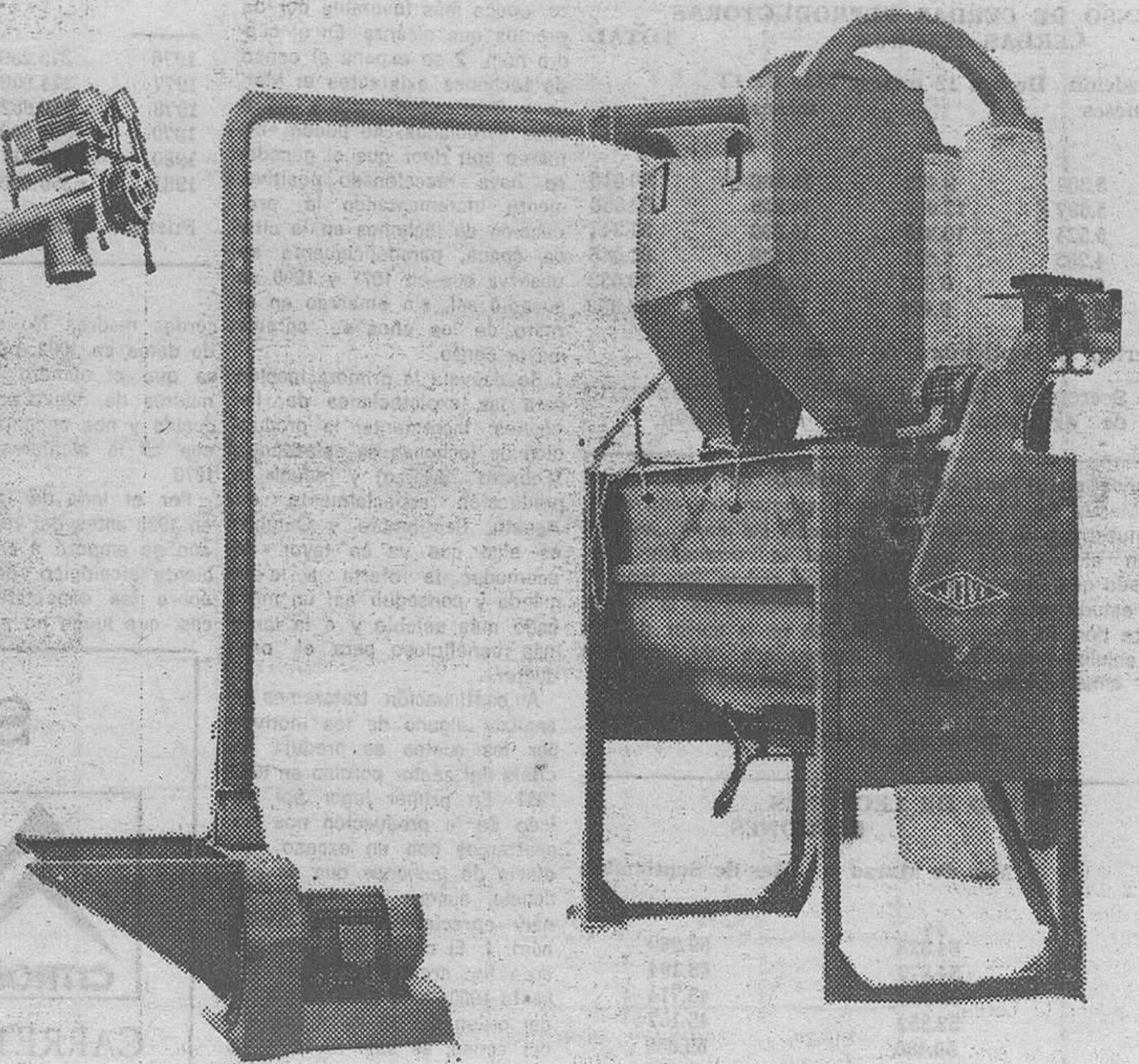
Conjunto de molino y mezcladora horizontal
