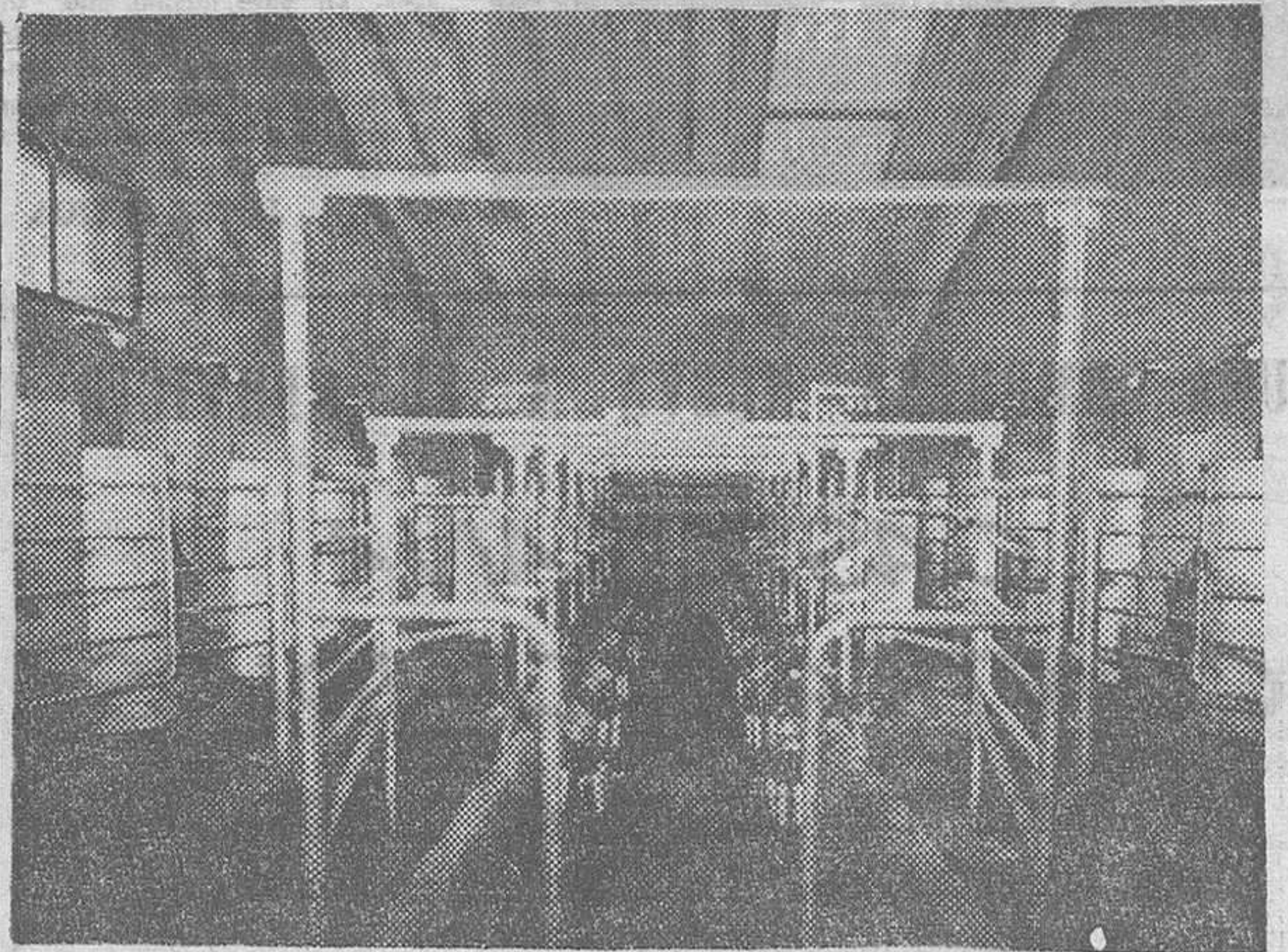
SALA DE ORDEÑO CON ACELERADORES EN POSICION DE LAVADO
