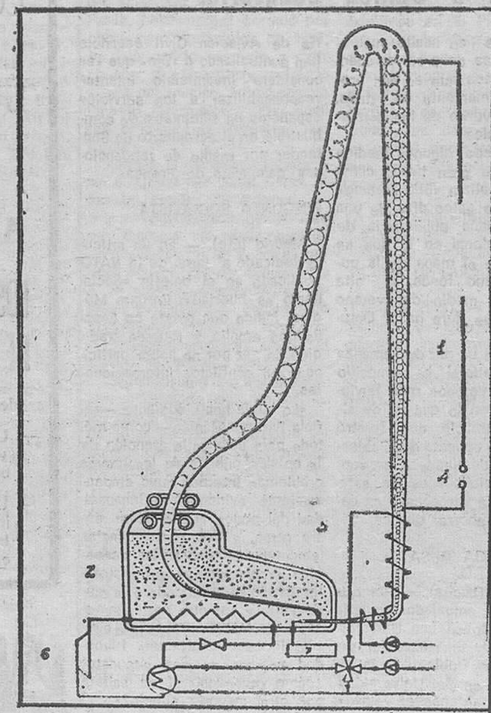
Esquema de la máquina termogravitacional de Diego Orellana: 1. — Columna de mercurio y generador eléctrico. 2. — Foco frío. 3. — Bola agente de transformación termodinámica. 4. — Salida de energía eléctrica utilizable. 5. — Foco caliente. 6. — Mantenedor del foco frío. 7. — Alimentación de las bolas a la columna de mercurio. — (Foto EFE-FIEL).
