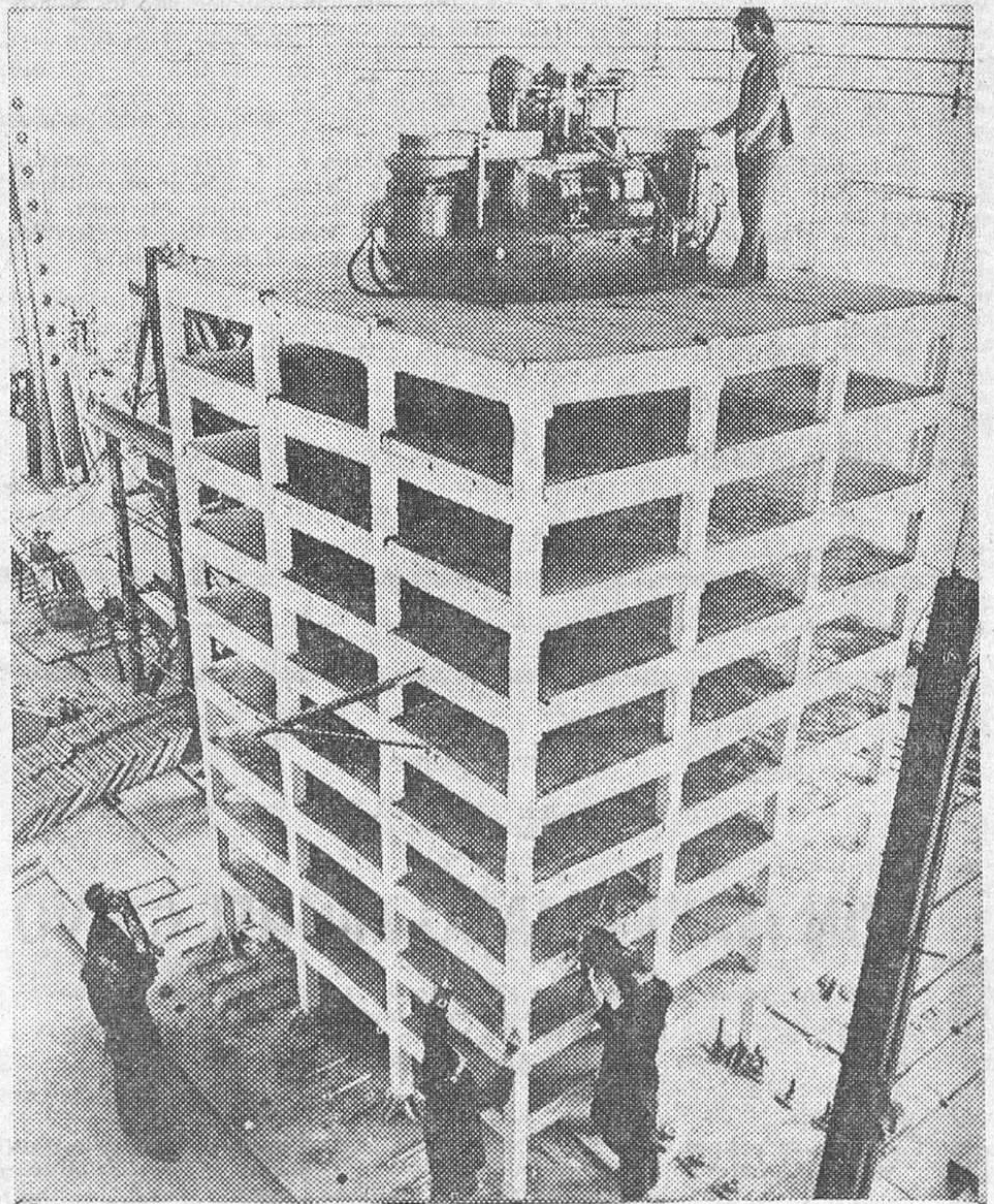
Todos los edificios de muchos pisos que se construyen en las repúblicas del Asia central, zona de actividad sísmica, reciben sacudidas de hasta nueve grados. Por ello, en la base experimental del Instituto Científico Zonal de proyección de edificios residenciales y públicos, en Tashkent, capital de Uzbekistan, los modelos de las futuras edificaciones se someten al efectos de "Terremotos" artificiales, como el que vemos en la fotografía. — (Foto FIEL).
