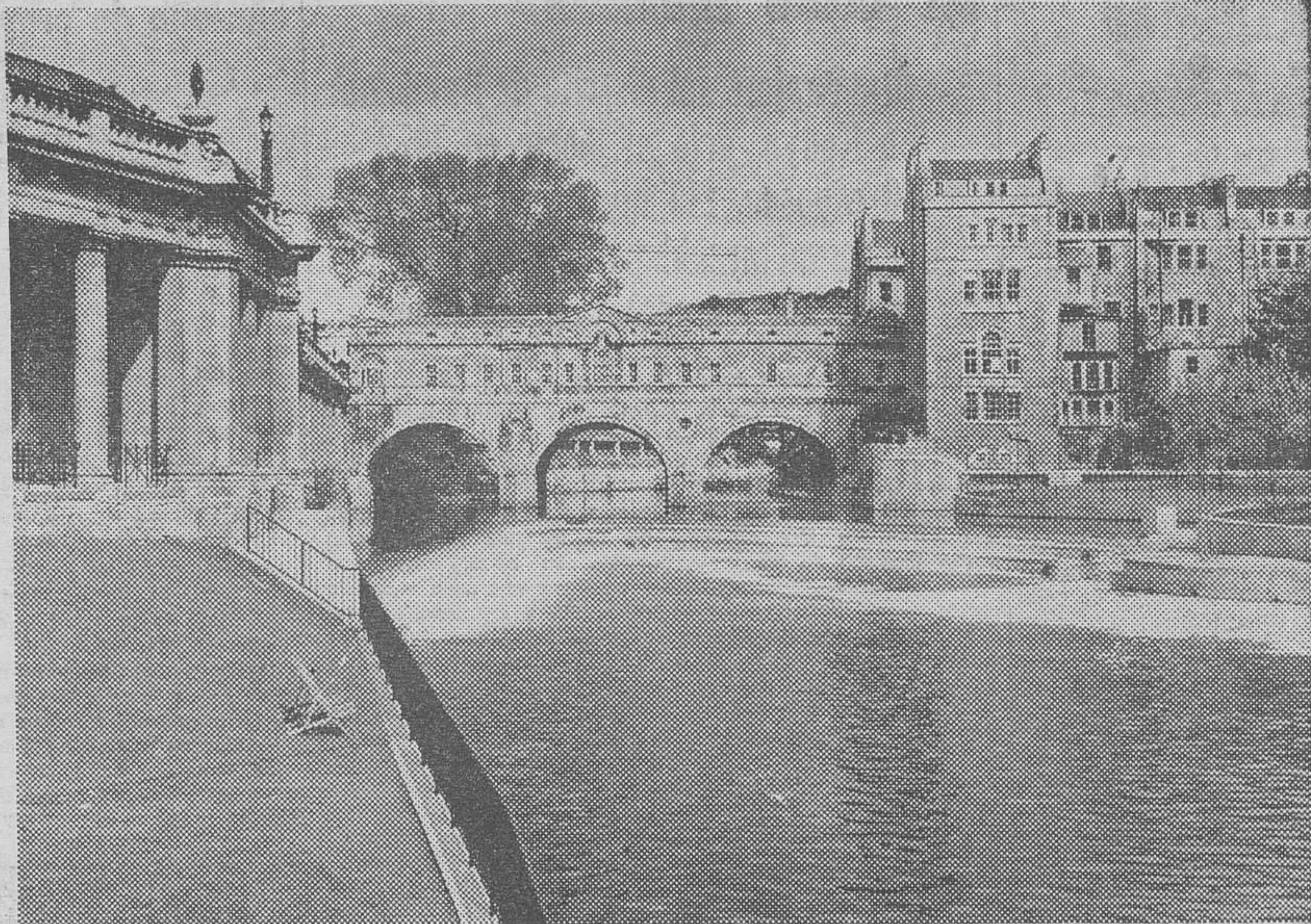
La reconstrucción de esta pequeña cuenca, en la presa de Pulteney, en Bath, antigua ciudad inglesa, ha obtenido el Premio 1972 del «Civil Trust». El trabajo ha sido efectuado como parte de un proyecto de protección contra las inundaciones, duplicado el caudal de esta sección del río Avon. Los arquitectos diseñaron para esta obra una compuerta, una isla con un pequeño atracadero de botes y un jardín en la orilla. El citado premio se concede en Inglaterra a todas aquellas obras o mejoras que ayudan a embellecer o a conservar el ambiente. — (Foto FIEL).
