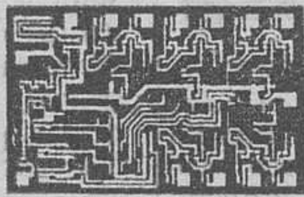
Microfotografía de un circuito integrado.
