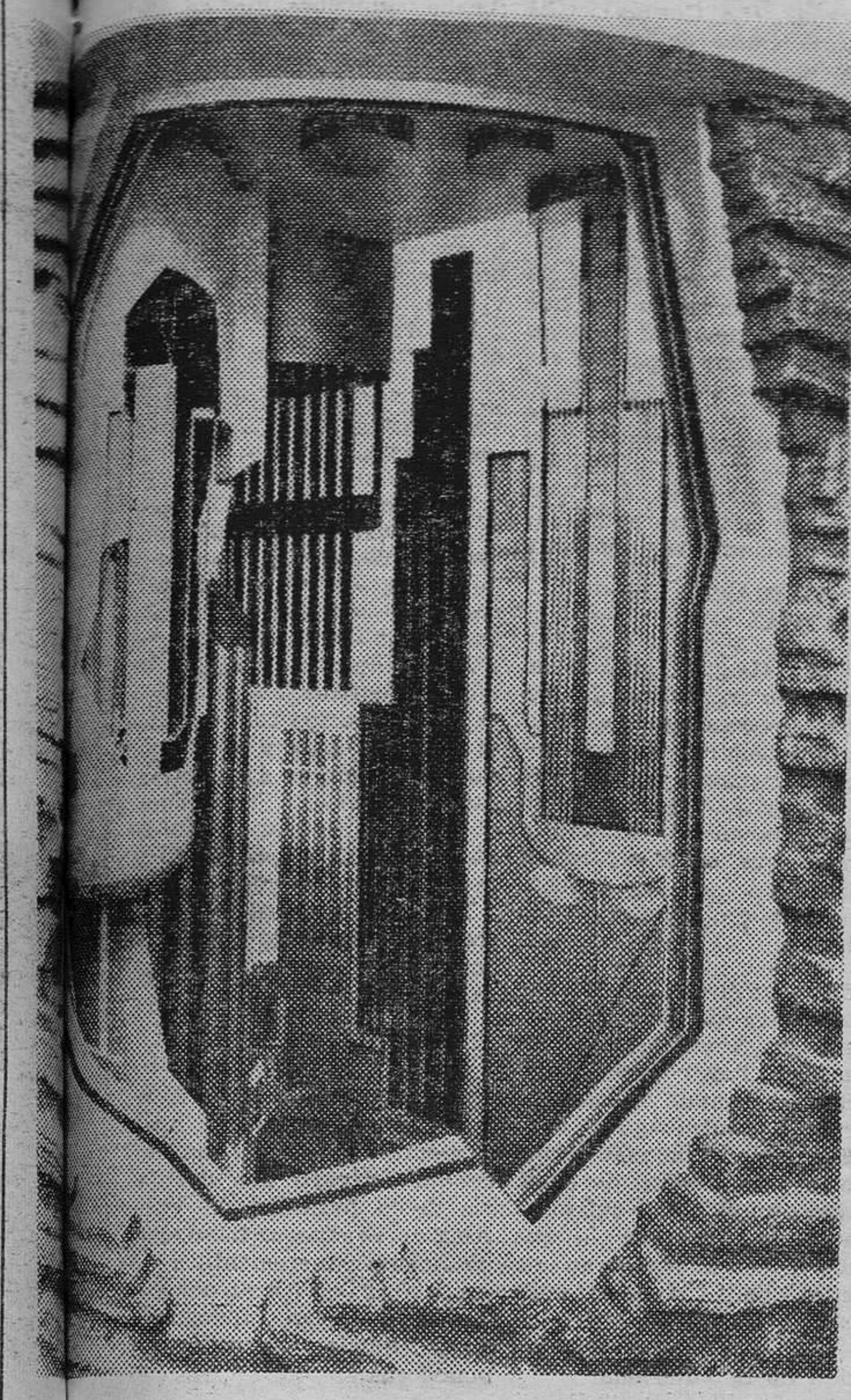
Este reactor rápido ha sido presentado por Gran Bretaña en la exposición «Ciencia y Paz», celebrada en Ginebra. Las características de este reactor construyendo en la ciudad escocesa de Dounreay, son: 2,1 metros de diámetro. El prototipo presentado en Ginebra presentaba un núcleo de uranio enriquecido con el 25 por ciento de 235 U, con objeto de ilustrar al visitante sobre su funcionamiento. — (Foto Fiel)
