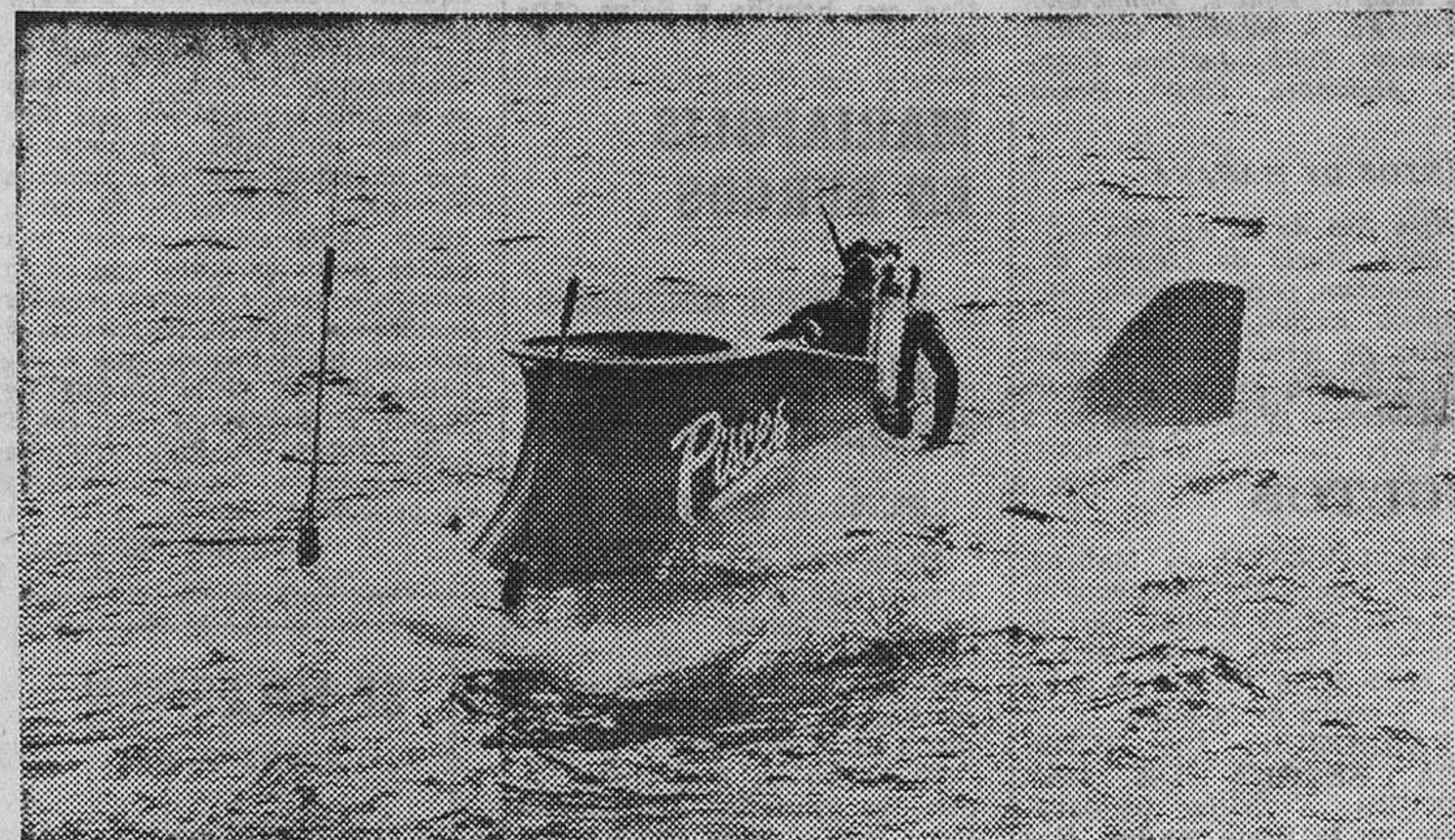
Este es el submarino especial monoplaça y de color amarillo, llamado «Pisces» (Foto CIFRA)
