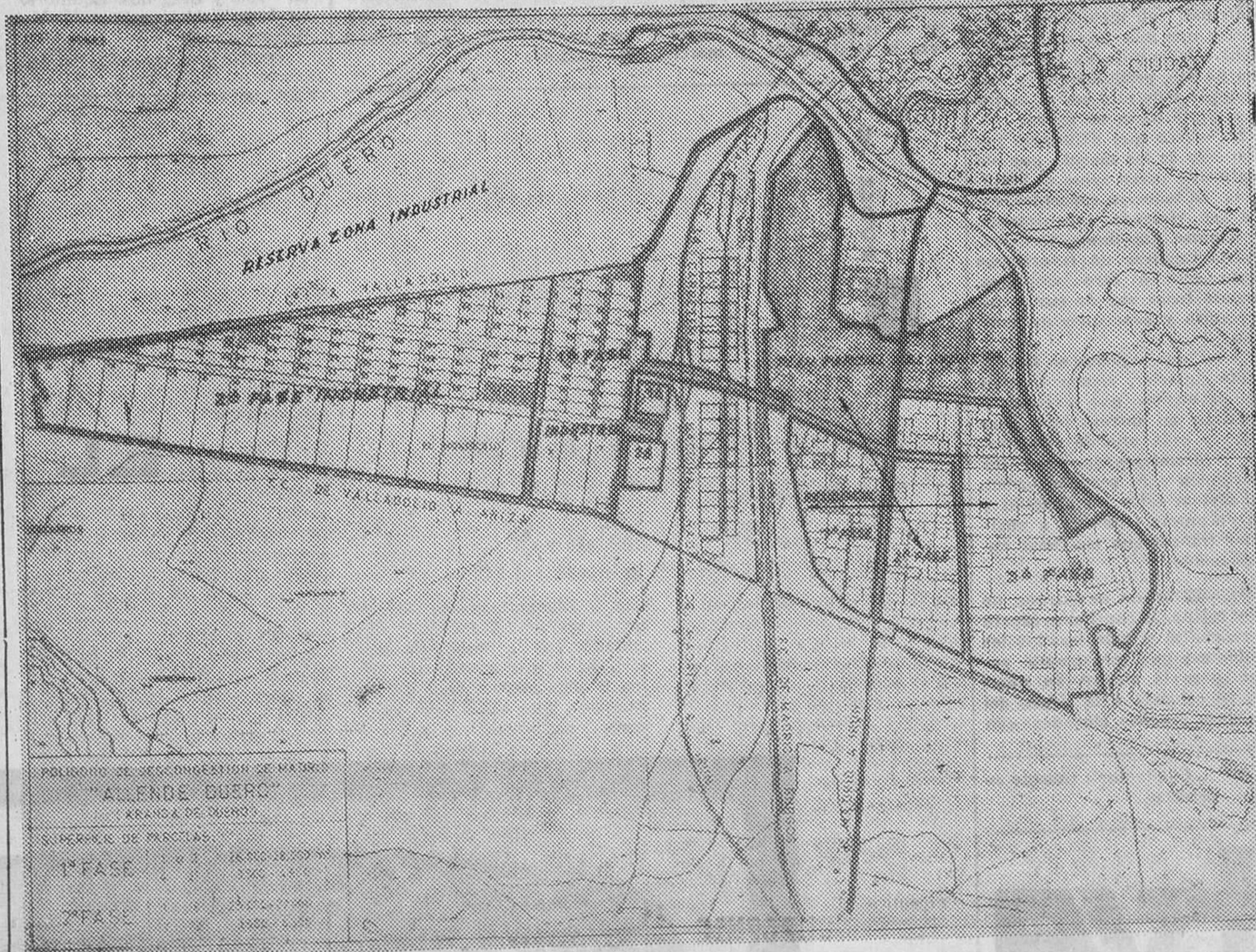
Fotocopia del plano de los polígonos industrial y residencial. El residencial está previsto para albergar una población de 86.000 habitantes
