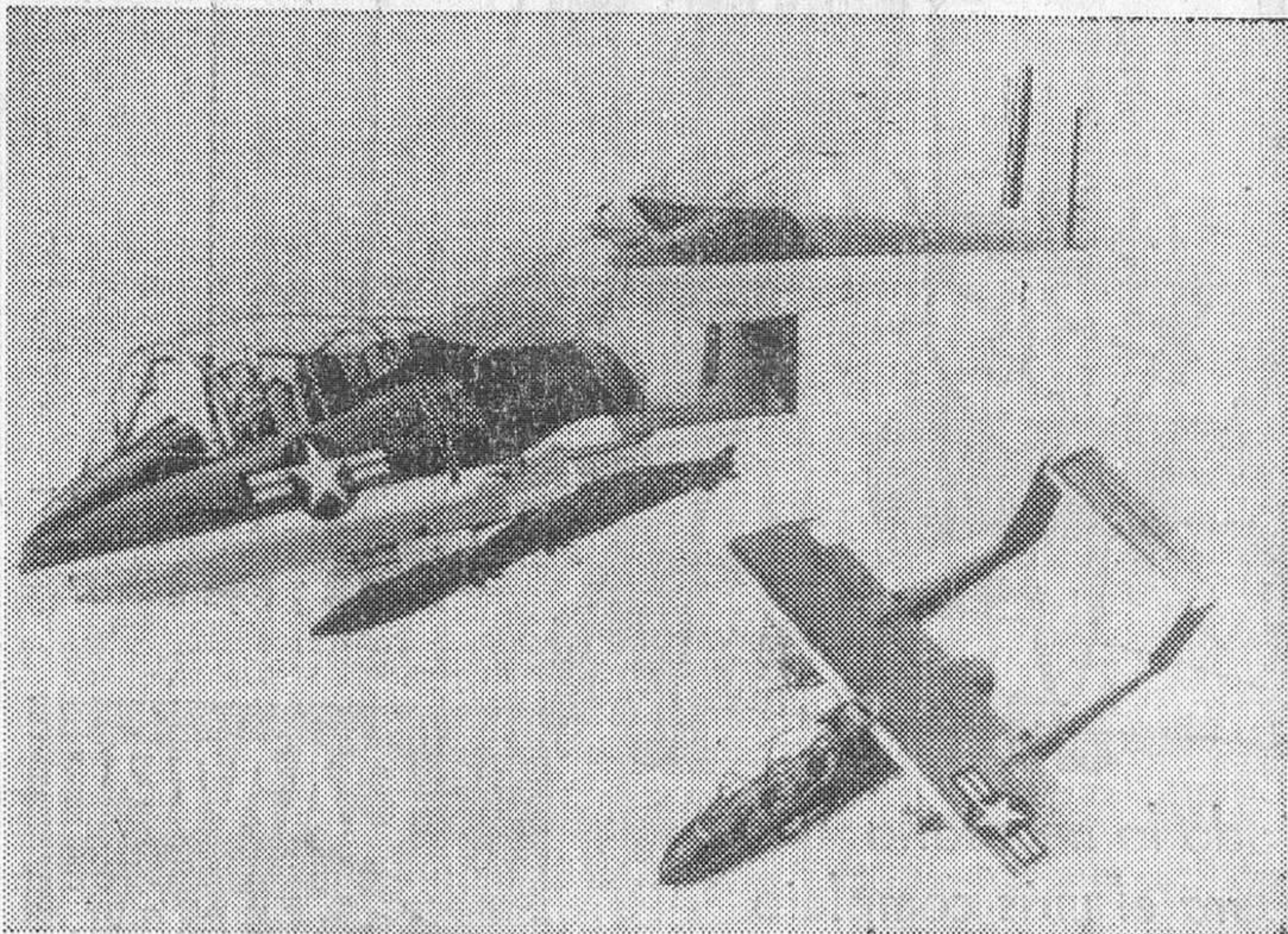
He aquí dos dibujos de un nuevo avión anti-guerrilla, que se halla en fase de realización en EE. UU. El presidente Johnson ha descrito este nuevo aparato como un "equivalente aéreo del jeep". El avión podrá realizar también funciones de emergencia en tiempo de paz, en caso de catástrofes y misiones médicas. Se espera que el aparato realice sus primeros vuelos en 1965. - (Foto Fiel).
