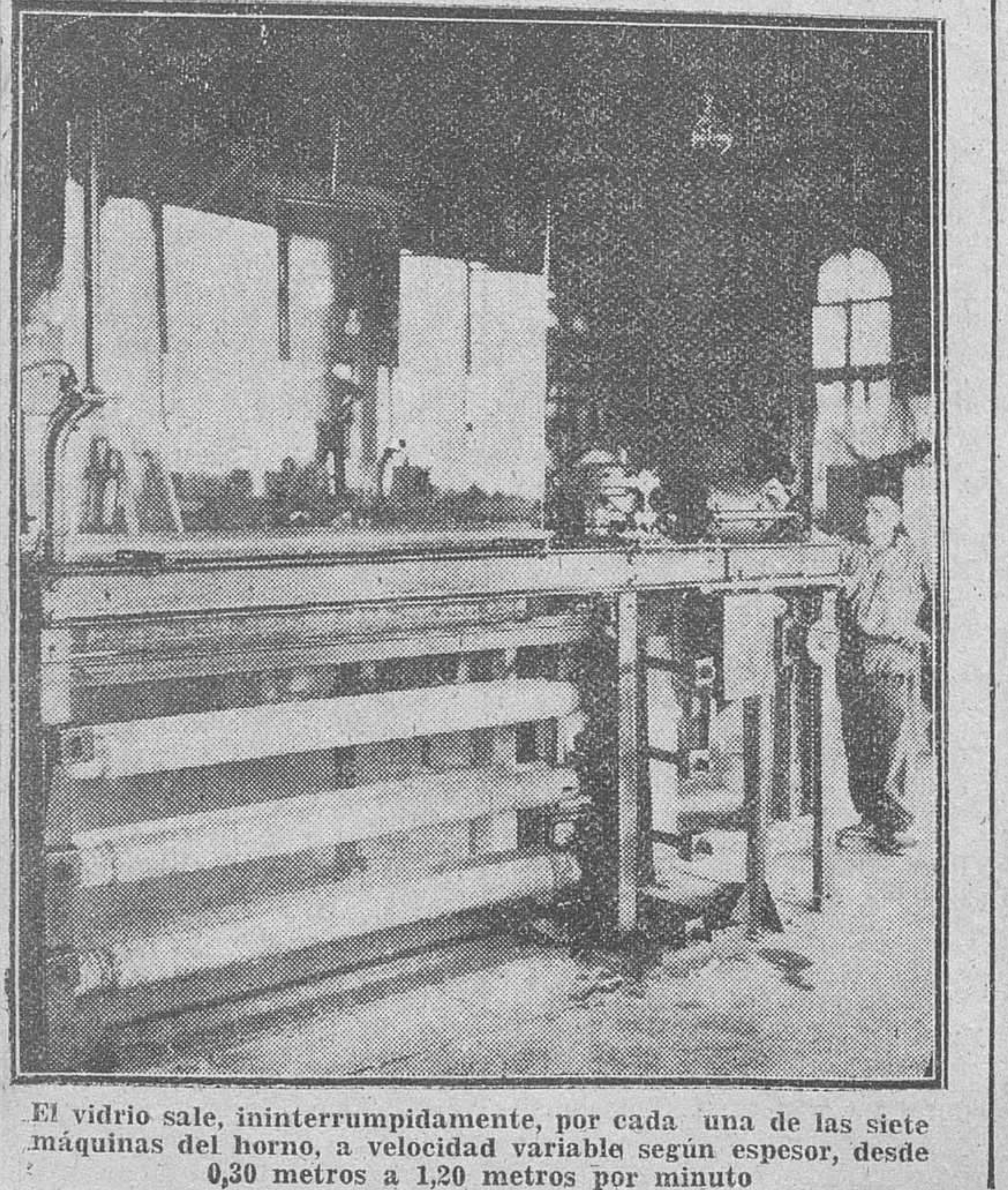
El vidrio sale, ininterrumpidamente, por cada una de las siete máquinas del horno, a velocidad variable según espesor, desde 0,30 metros a 1,20 metros por minuto.
