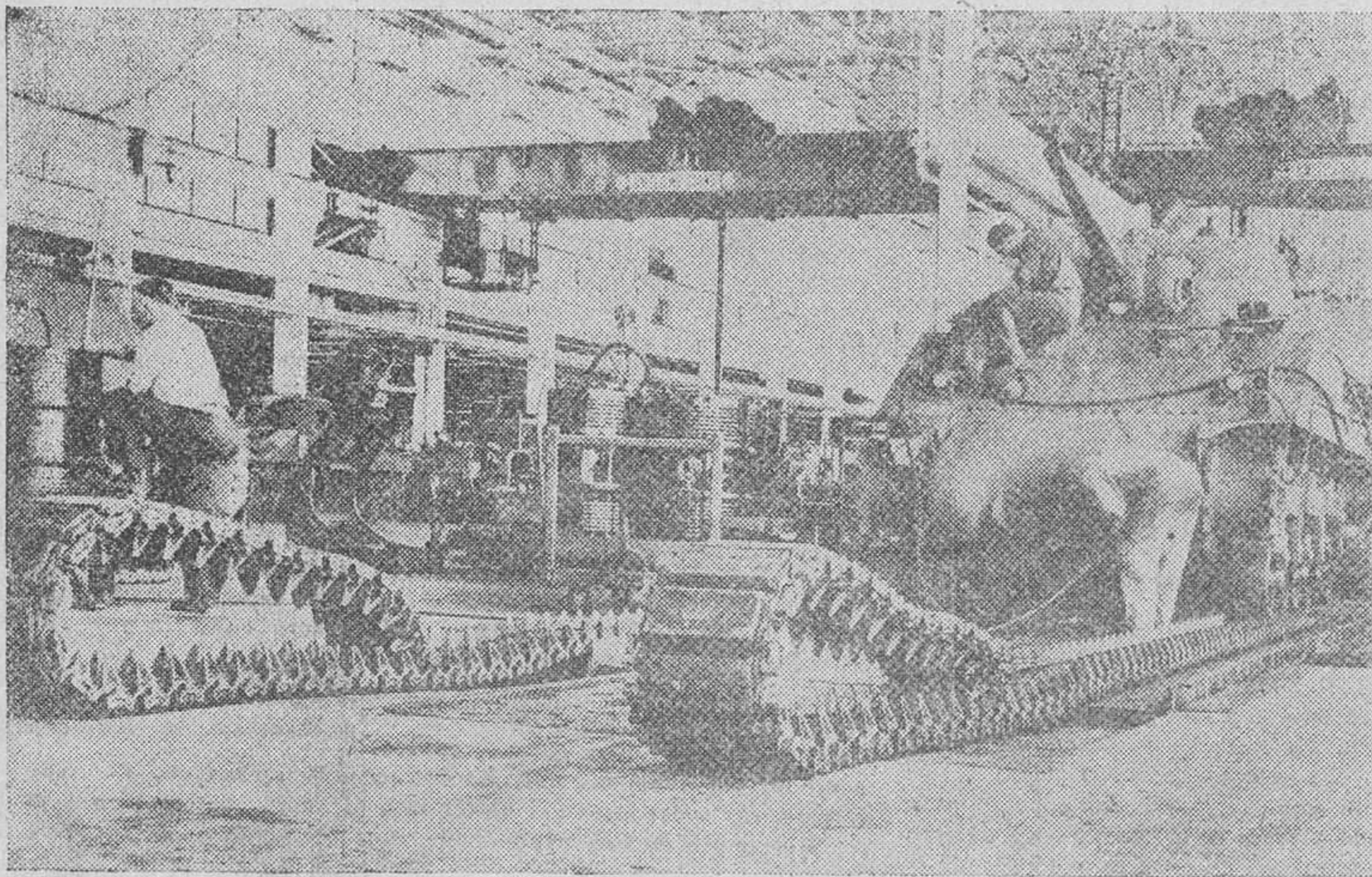
Estas fotos representan escenas tomadas en una gigantesca fábrica de guerra de la zona central de los Estados Unidos, que construyó en serie durante la guerra tanques soldados, en tres cadenas de producción. Una de las operaciones más espectaculares de la fabricación del gigante de 30 toneladas es el tendido de las orugas para el M-4, como nos presenta la foto.
