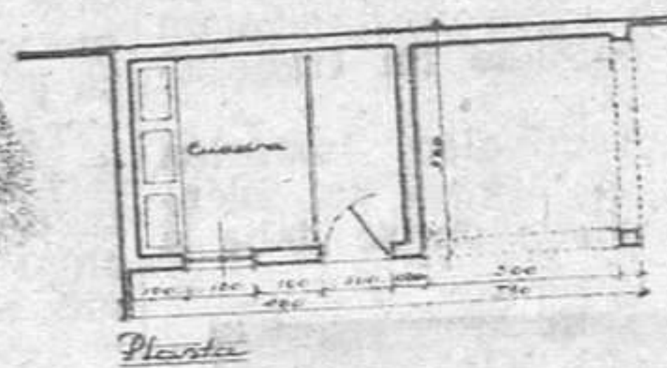
Planta
