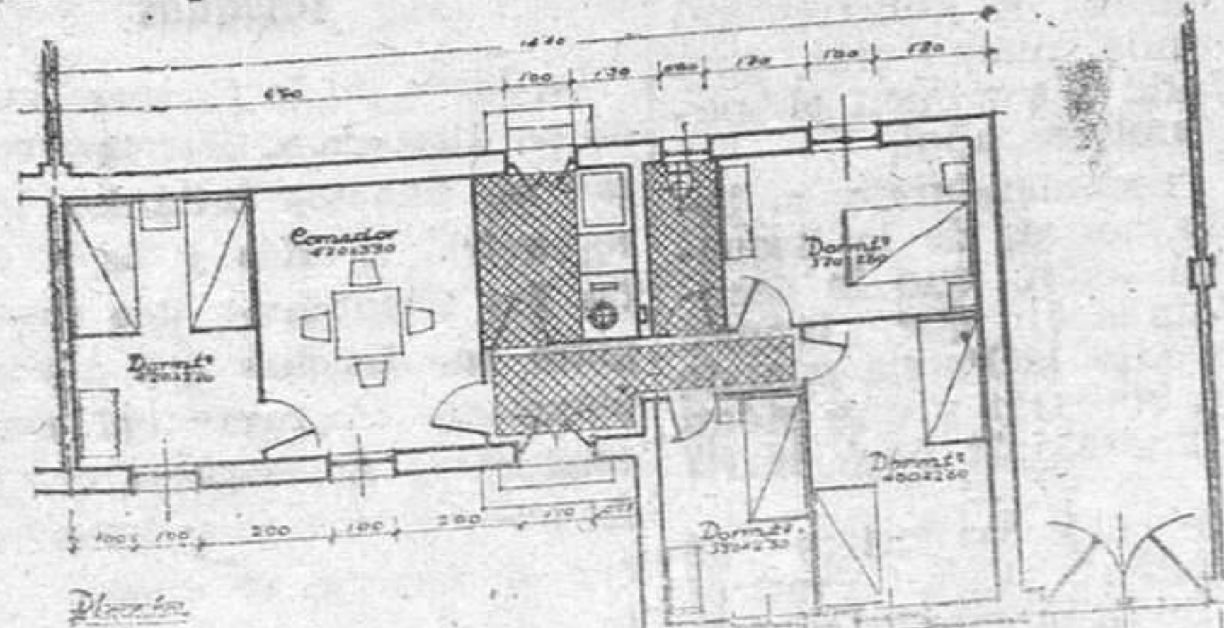
Planta
