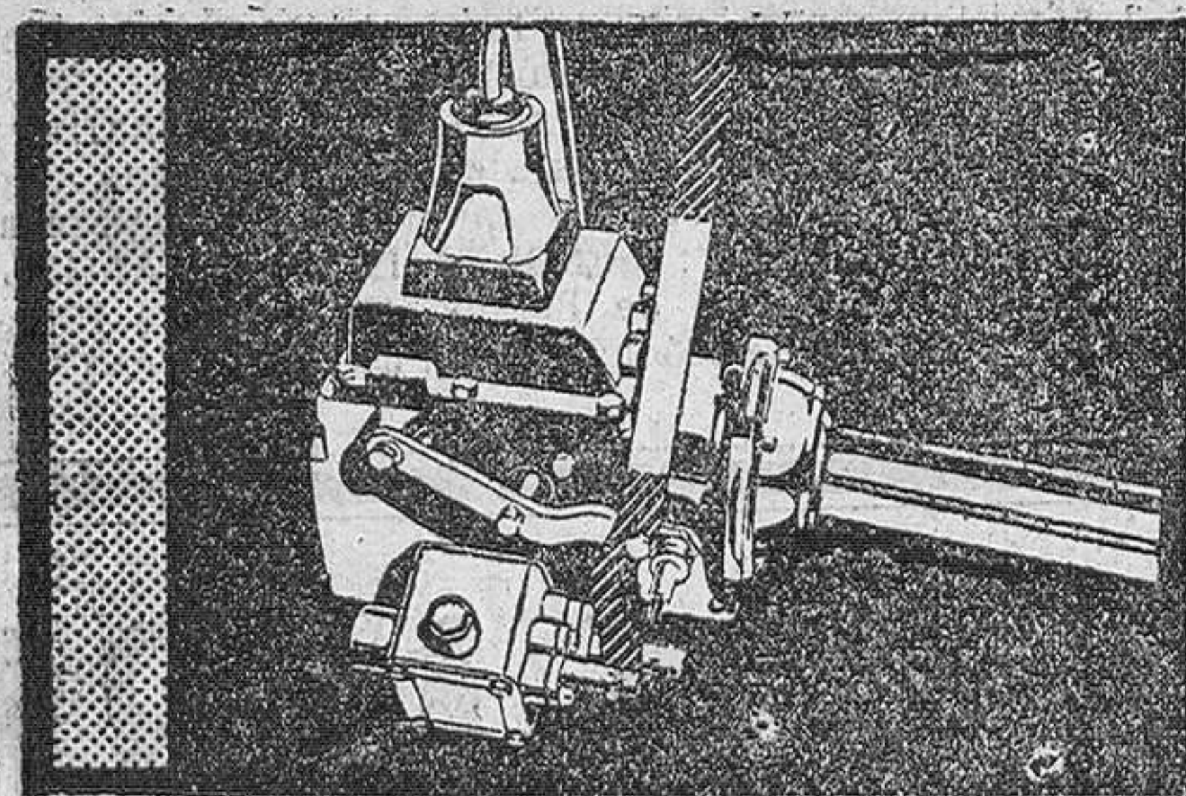
Caja de cambios de cuatro velocidades, que aumenta el rendimiento del camión. A la caja de cambios se puede acoplar una toma de fuerza para aplicarla a cualquier uso industrial
