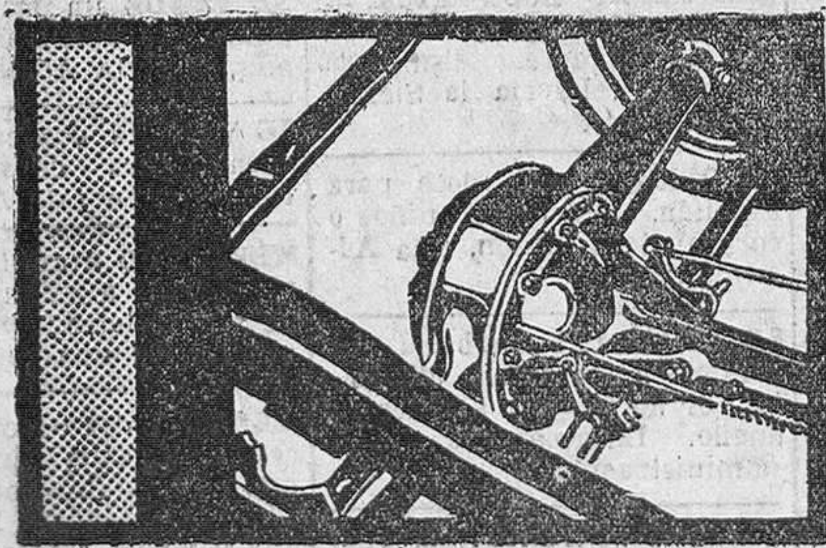
El nuevo eje trasero está encerrado en una sólida cubierta, provista de una tapa, que permite inspeccionar y ajustar el eje sin desmontarlo
