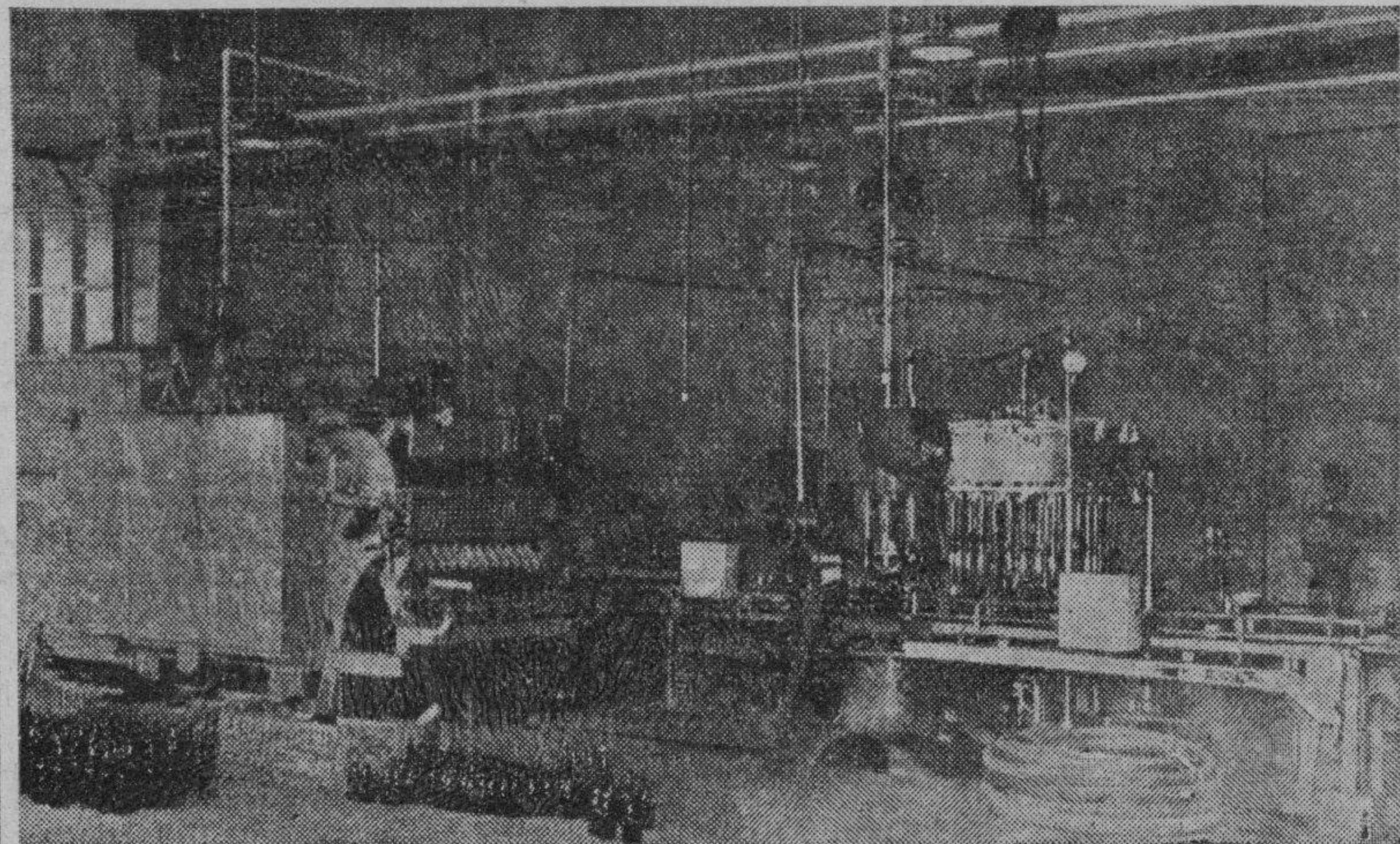
Como "nace" una botella de cerveza. La maquinaria intrincada que embotella las bebidas en la fábrica de Balintawak. La máquina a la izquierda limpia la botella, que va después al rellenador, donde la cerveza se vacía en un recipiente, y luego finalmente, al colocador de la tapa, donde la botella se cierra.
