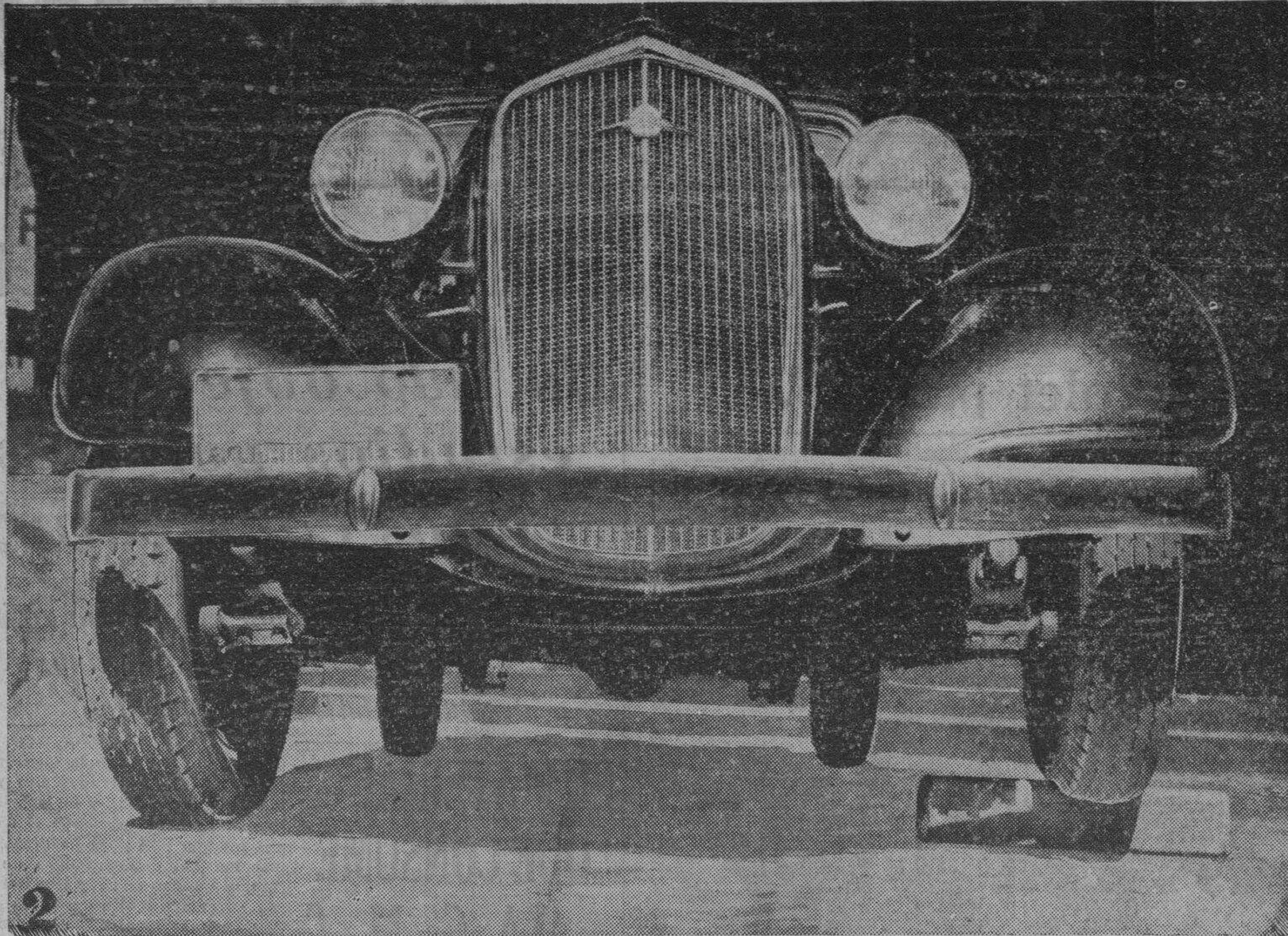
El nuevo modelo del Chevrolet para 1934 visto de cerca para mostrar la disposición del eje delantero con la mas reciente mejora de ruedas con efecto de rodillas. Como se ve en esta fotografia los muelles que permiten un movimiento independiente para cada rueda están bien cubiertos para protegerlos contra el polvo y agua. El efecto de los es los sorprendente, y como se ve en la fotografia la rueda puede pasar por sobre un objeto mas cénado que el nivel del camino sin que se sientan sus efectos por los pasajeros ni causar la inclinación del coche.
