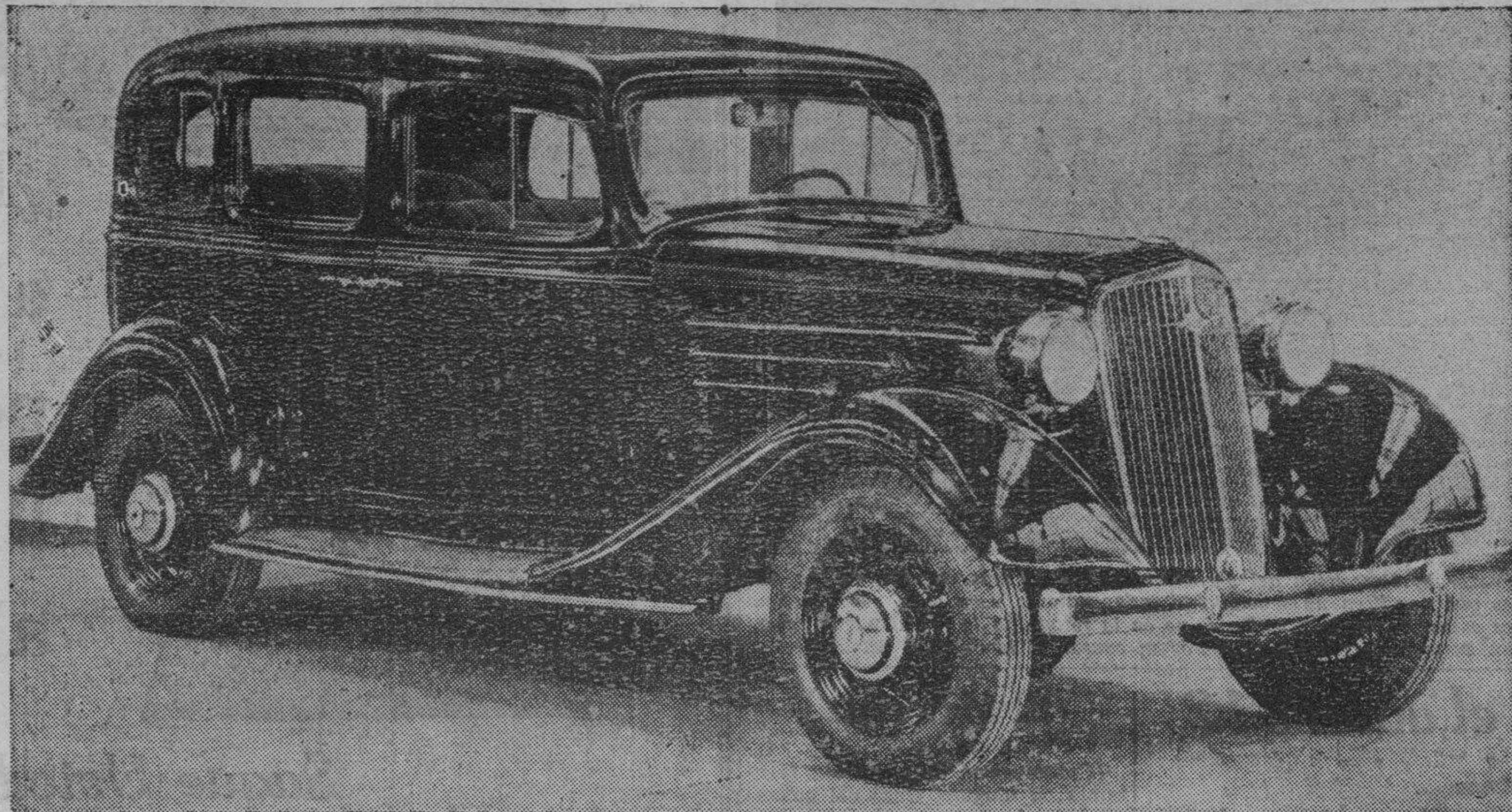
La fotografia muestra el primer Chevrolet Seis de 1934 que llegó a Filipinas. Tiene el volante en el lado izquierdo. Fue usado durante varias semanas para demostrar las ruedas de efecto de "rodillas" a los que estén interesados en este adelanto importante. Algunos modelos de sedan, coupé y town sedan, están ahora en exhibición. Solo se necesitan cinco minutos para saber lo que significan las ruedas de efecto de "rodillas" desde el punto de vista de la suavidad en la marcha y en las mejoras mecánicas.
