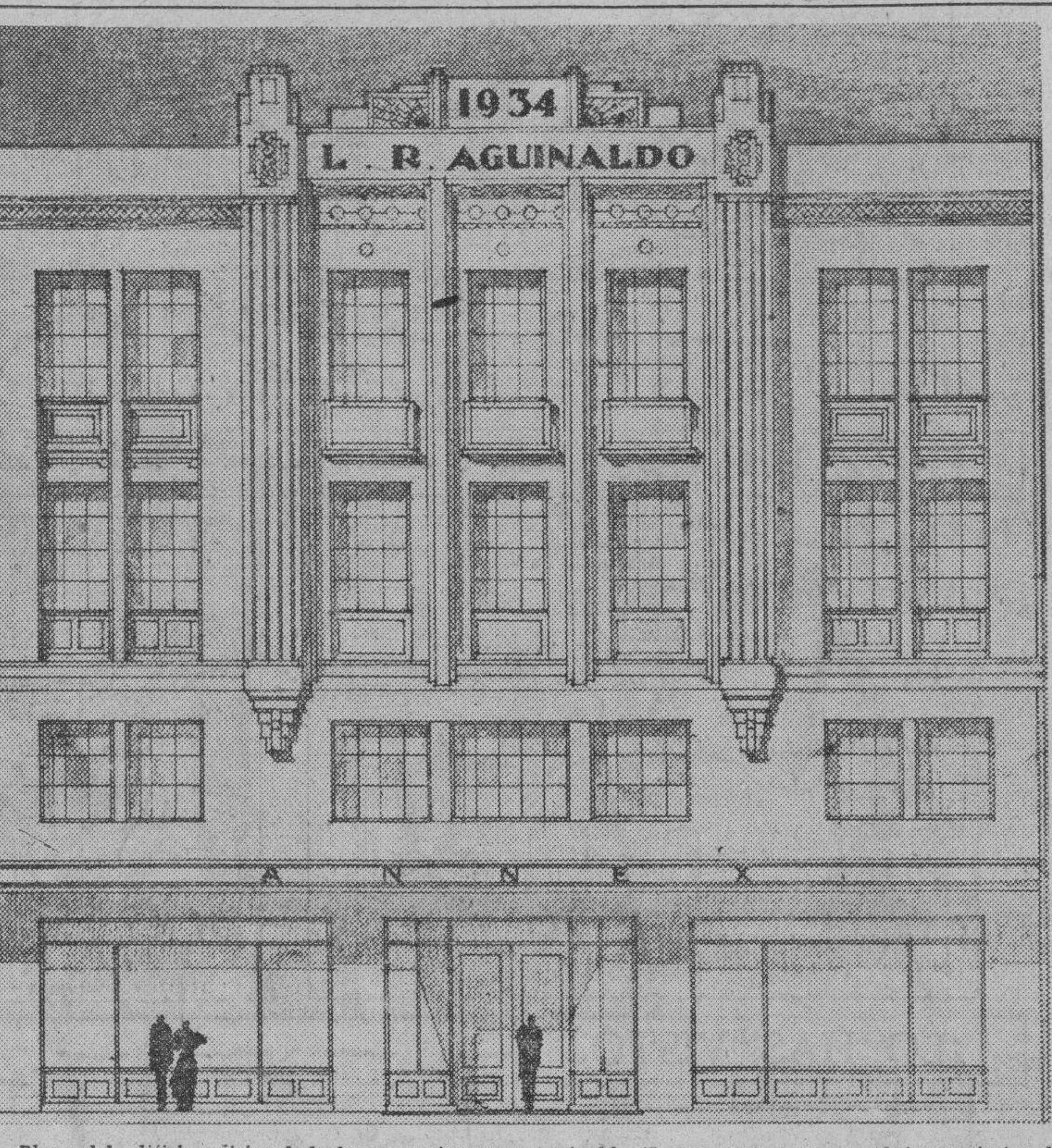
Plano del edificio adicional de la progresiva casa Aguinaldo (L. R.) para el cual se abrieron ofertas de contratistas el día 25 de agosto. El edificio ocupará un área de 153 metros cuadrados, tendrá un ascensor y un cuarto de fumigación y laboratorio químico.
