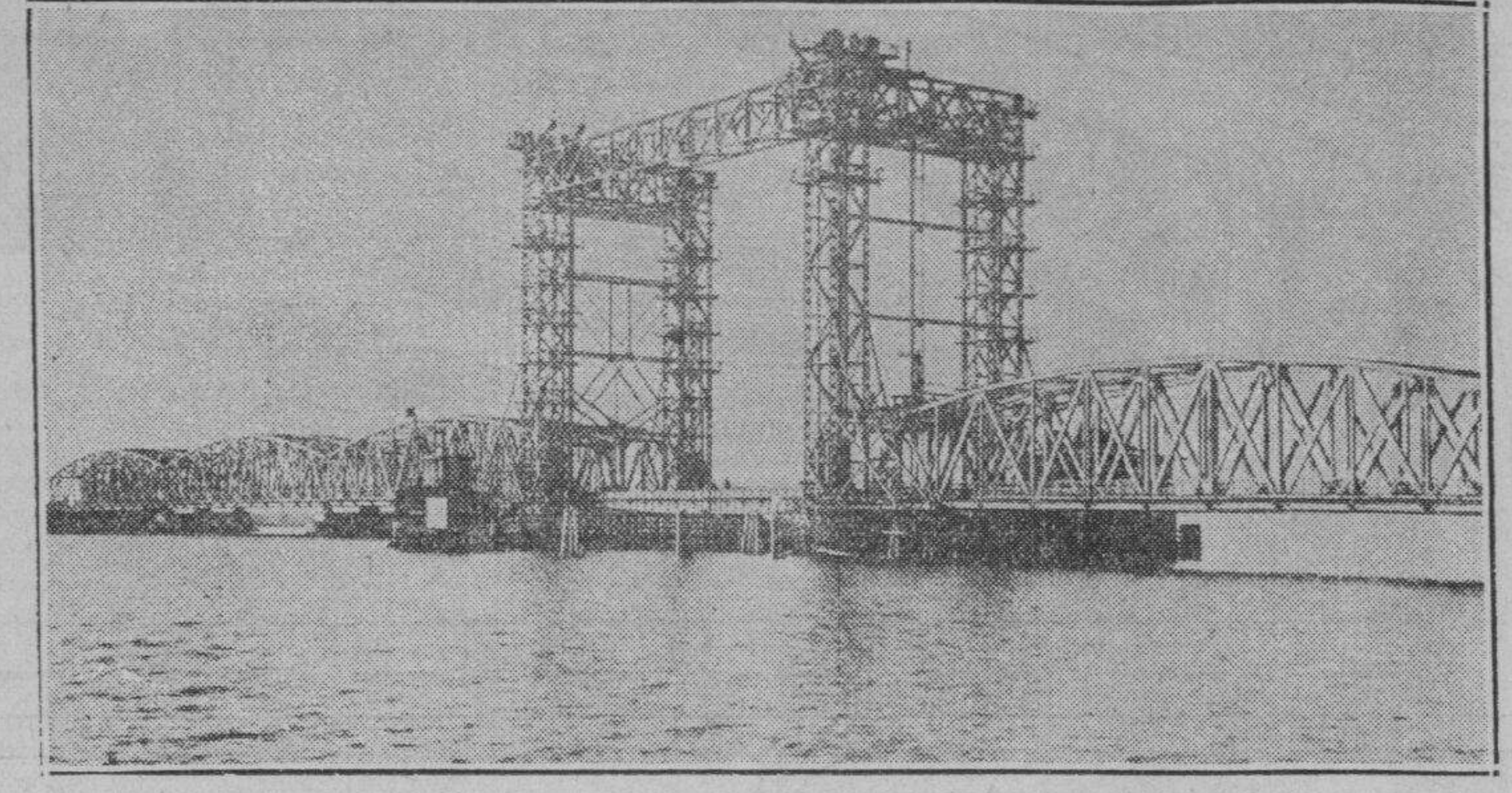
Una nueva idea en la construccion demuestra este puente que atraviesa el rio Peene, cerca de Karnten, Alemania. La seccion central del puente esta construida de tal forma que permite el paso de lanchas. Esta parte es levadiza, y se opera al estio de un ascensor.
