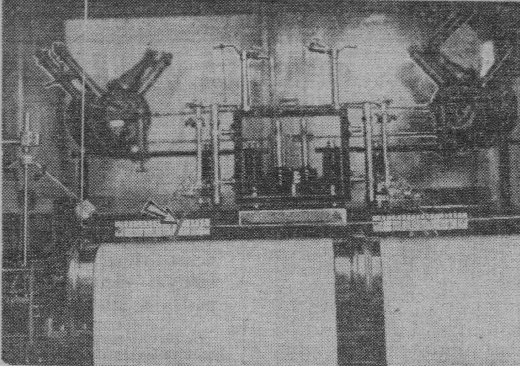
Fotografía tomada del instrumento sismográfico del Observatorio que ayer tarde registró el temblor que sacudió la ciudad y varias provincias. La flecha señala la aguja que saltó más allá de sus límites, impulsada por la fuerza del temblor.
