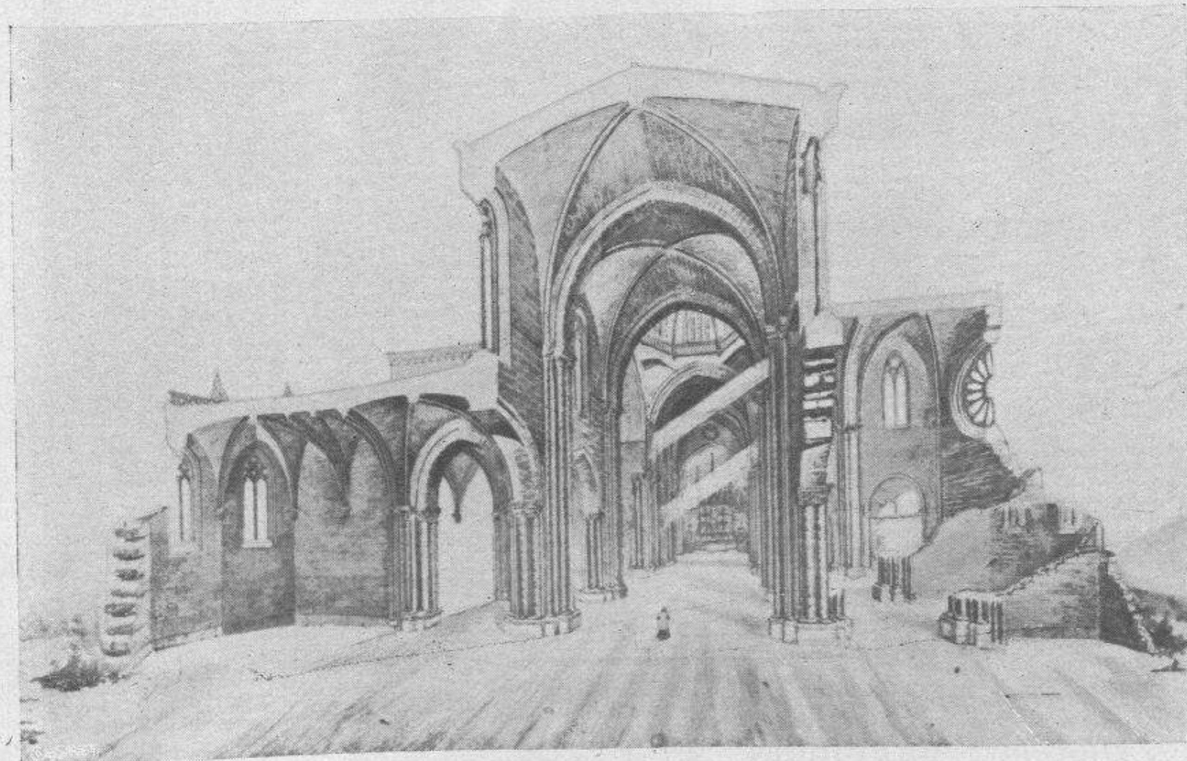
Catedral : Sección — Coupe.
