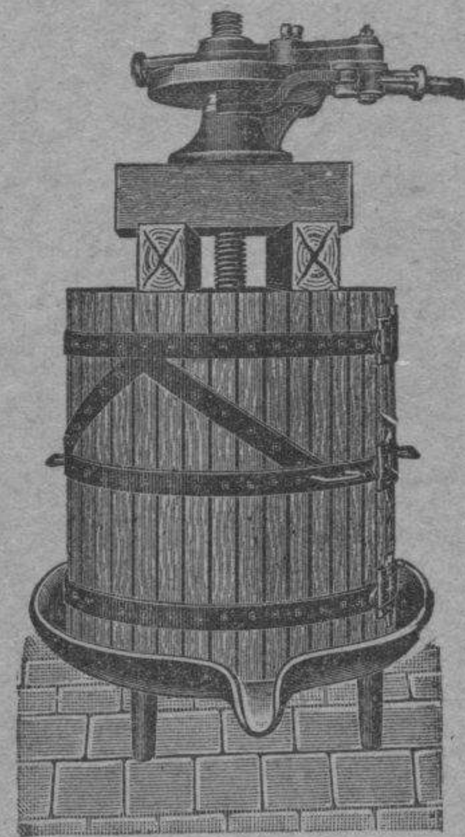
Presna para vino, de especial construcción, de AVERLY, S. A.
