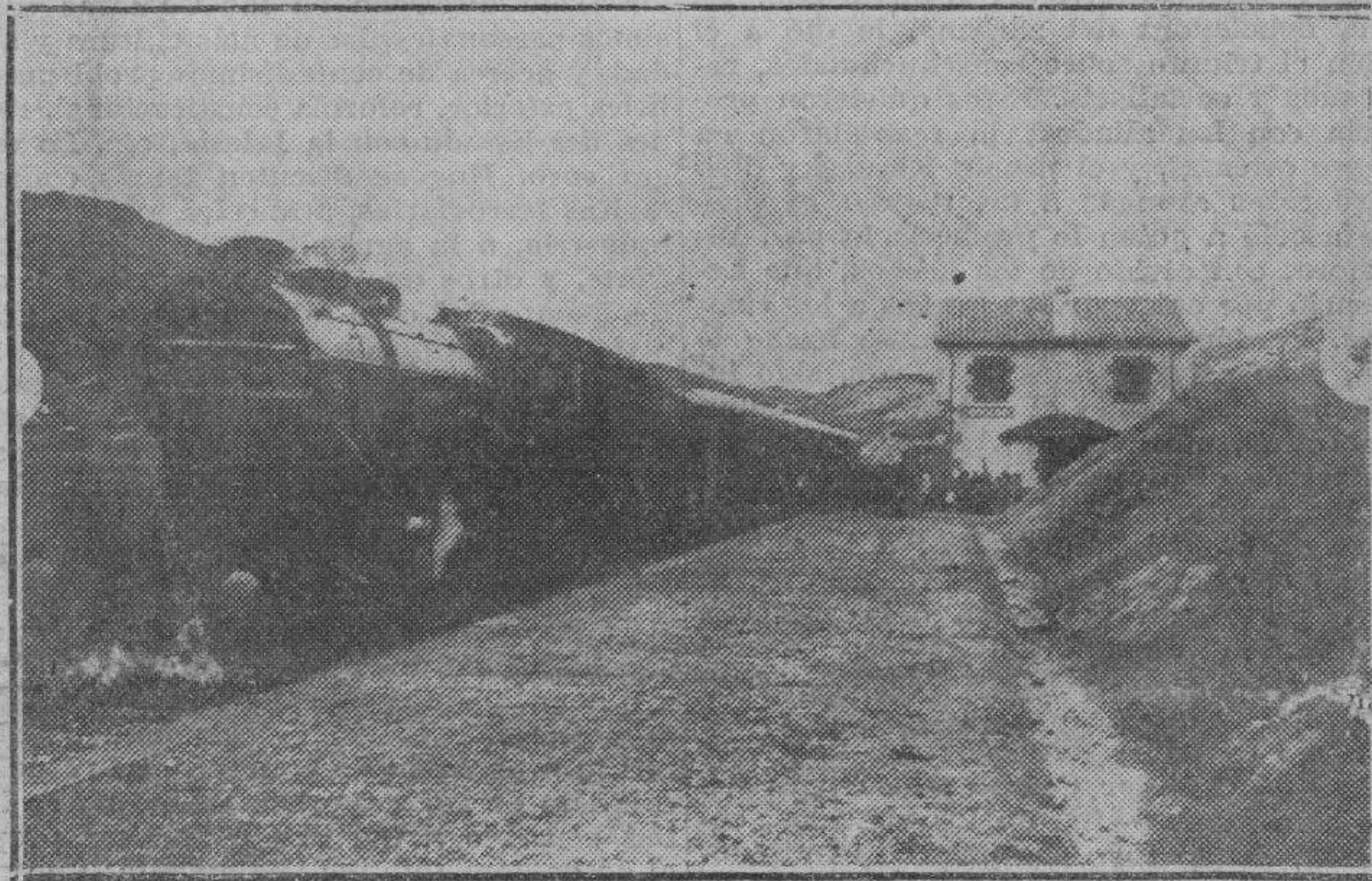
CALATAYUD.—Tren en Torrelapaja, que condujo a los invitados a la inauguración del trayecto de Calatayud, en el ferrocarril Santander-Mediterráneo (Foto. Rubio)
