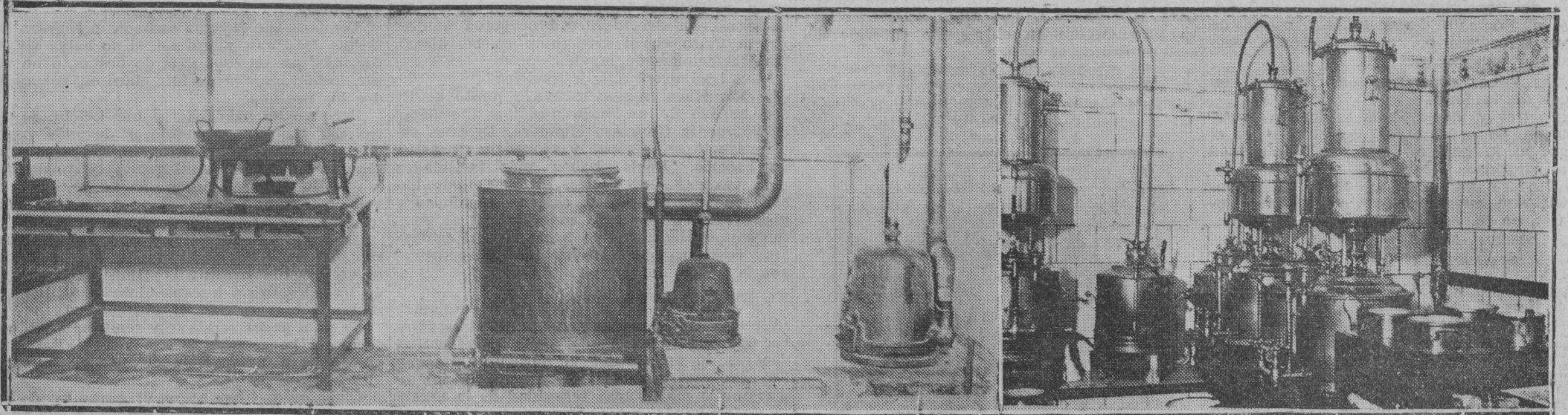
CASINO MERCANTIL.—Gran cocina a gas, distribución de agua caliente y servicios de cafetería a gas para 700 servicios
