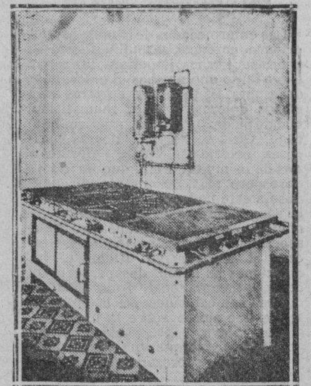
POLITECNICA TORRES.—Gran cocina a gas para 200 raciones y distribución de agua caliente
