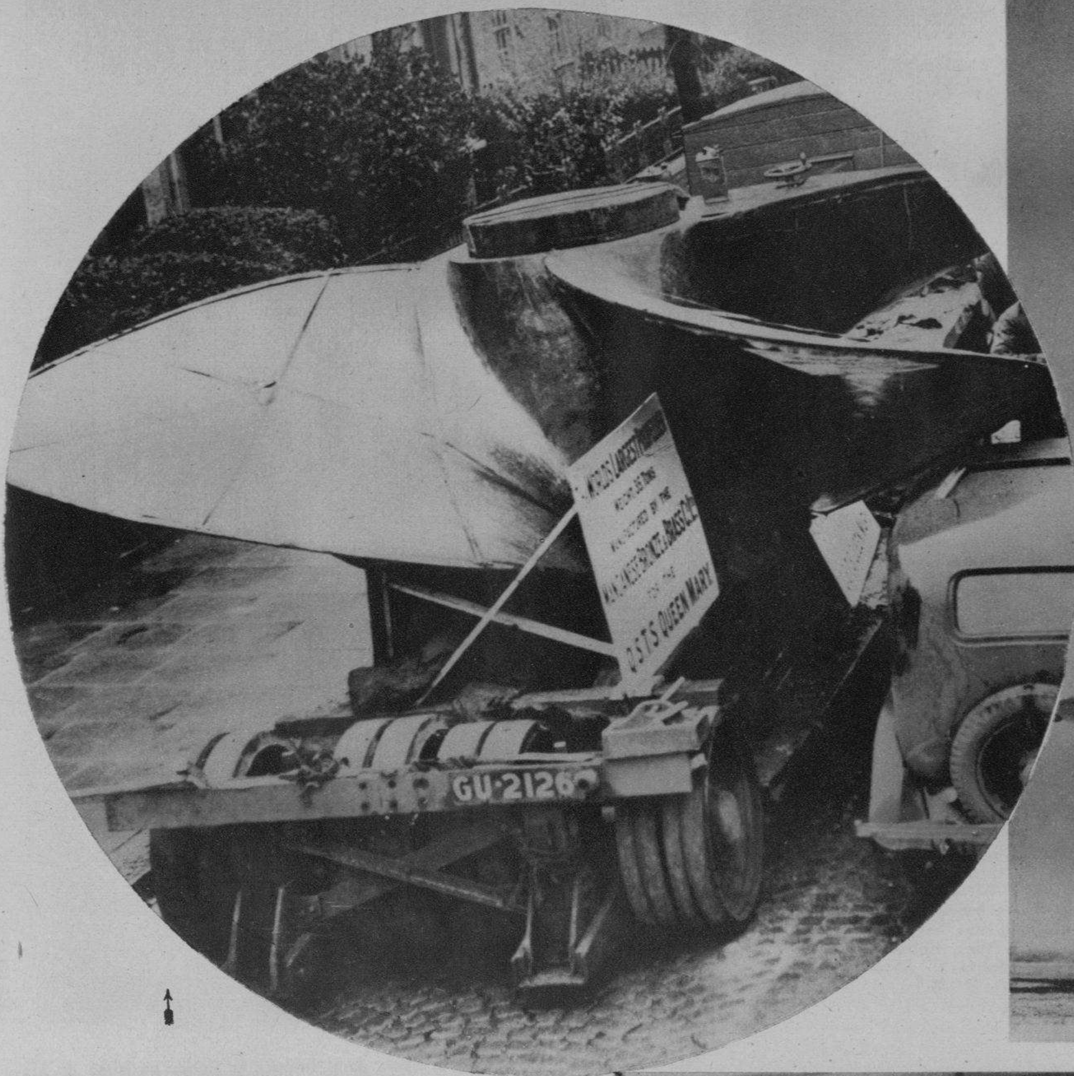
UNO DE LOS propulsores del "Queen Mary", el nuevo gigante de la Cunard White Star Line, que iniciará sus viajes pronto, pesa 35 toneladas. Ha sido construido en Milwall (G. Bretaña) y se exhibió antes de ser transportado a Southampton para su instalación (Foto Wide)
