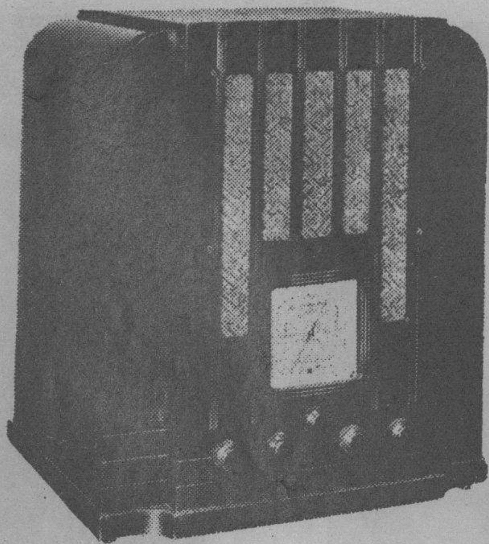
Modelo M-81 - 8 TUBOS Recibe ondas de 16 a 2000 metros
