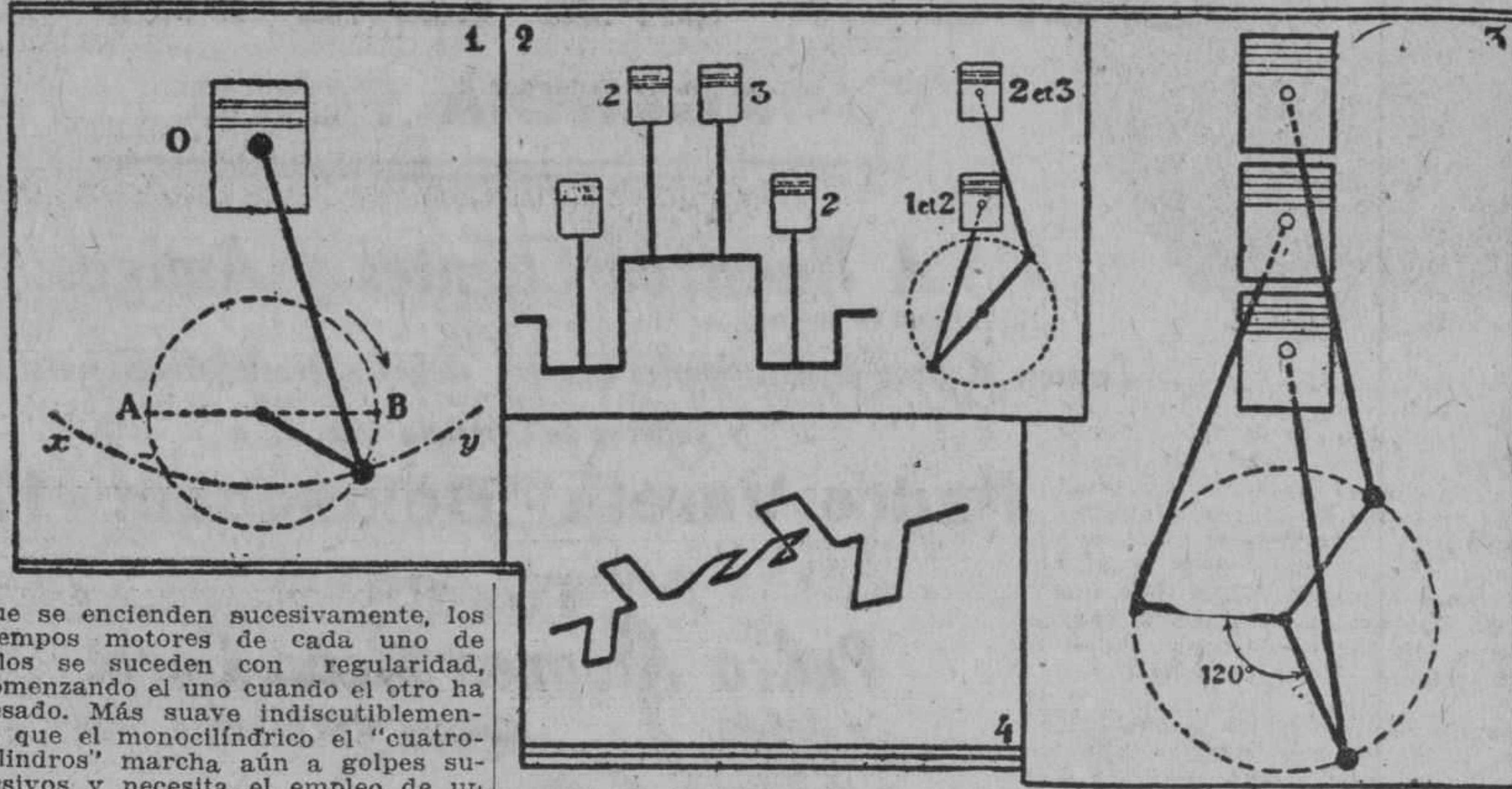
Fig. 1: En cada momento, la articulación biela-cigüeñal, se encuentra sujeta a detenerse sobre dos codos diferentes; el círculo AB descrito por el cigüeñal, y el arco xy de rotación instantánea de la biela alrededor de O. Según la posición del pistón, según que el cigüeñal describa el arco AB o el arco BA, estos dos movimientos son, o semejantes o en oposición; y resultan de ello esfuerzos irregulares en todo el conjunto. Fig. 2: Simétrico, el "cuatro cilindros" no goza más que de un equilibrio aparente. En razón de la oblicuidad de las bielas, las velocidades lineales de los pistones que suben y bajan, son diferentes en cada momento; por consiguiente, el centro de aplicación de las fuerzas varía continuamente. Fig. 3: Esquema en corte del equilibrio espontáneo de las fuerzas de inercia de un "seis cilindros". Fig. 4: El árbol cigüeñal de "seis cilindros", contrariamente al de cuatro es de una fabricación bastante compleja; sus codos están orientados en tres planos inclinados a 120°.
