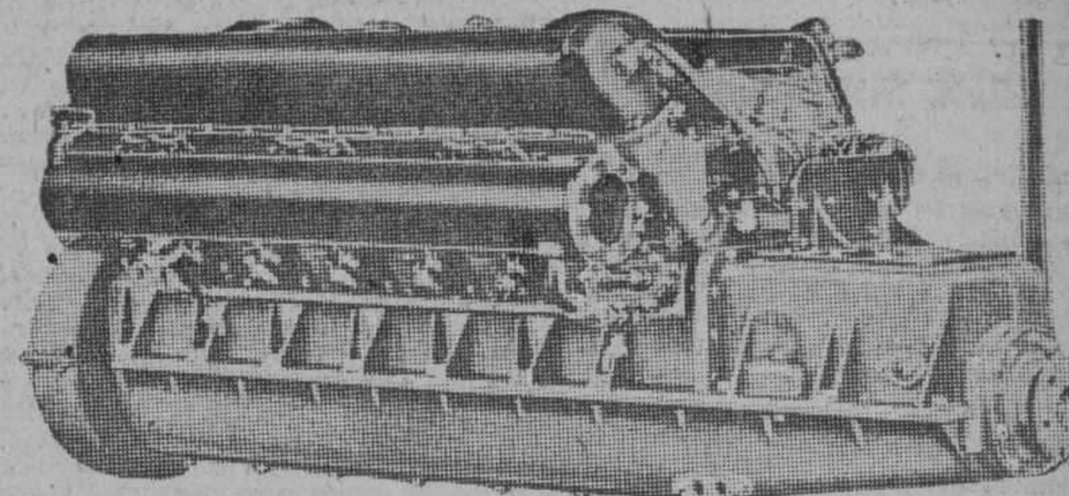
Motor Packard 12 cilindros de los botes vencedores del Campeonato de 150 millas en 1927 y 1926 y de otros grandes trofeos.
