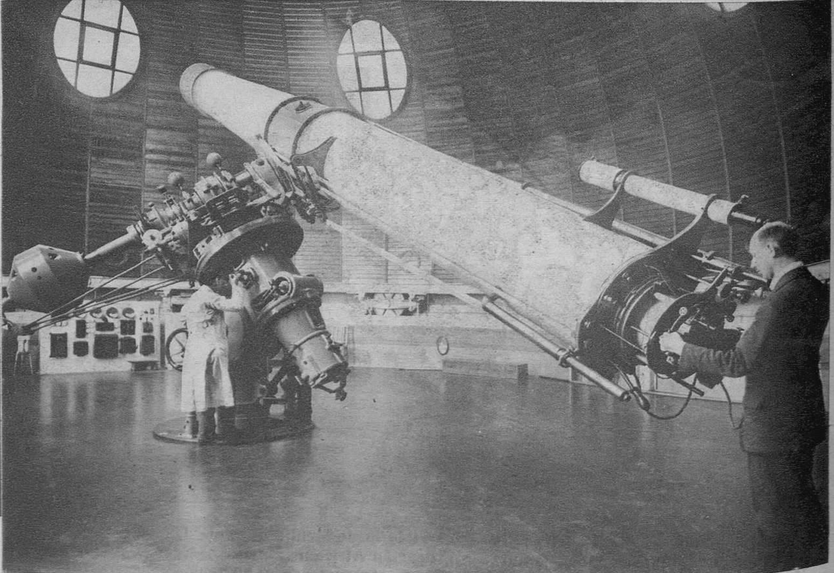
Una vista de la sala del observatorio de Sternwarte de Berlín, con su gigantesco telescopio de 65 cm. de diámetro, y que por una colocación especial puede ser movido en todos sentidos. (Foto Martín)
