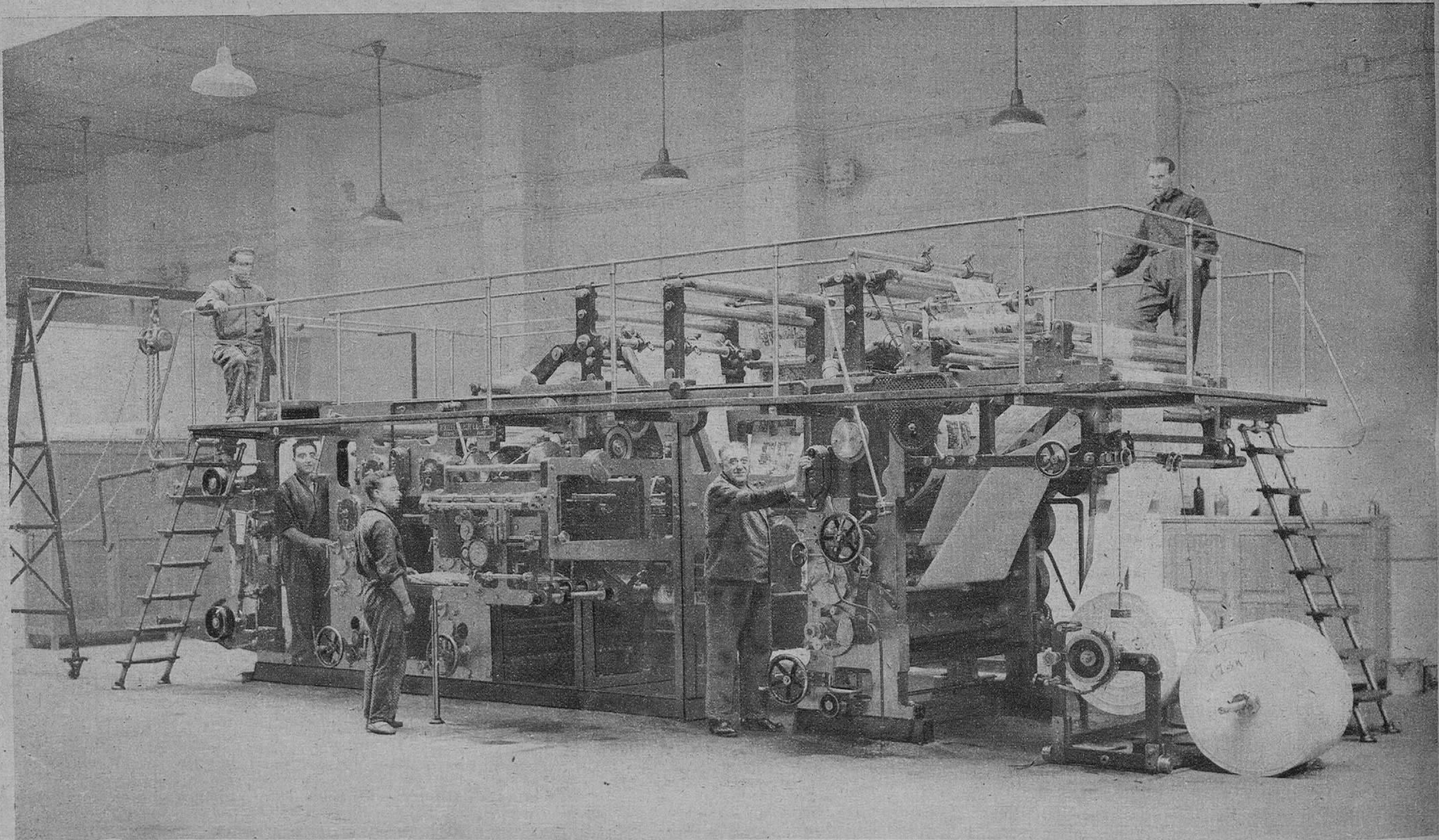
Máquina rotativa para impresión tipográfica y huecograbado.
