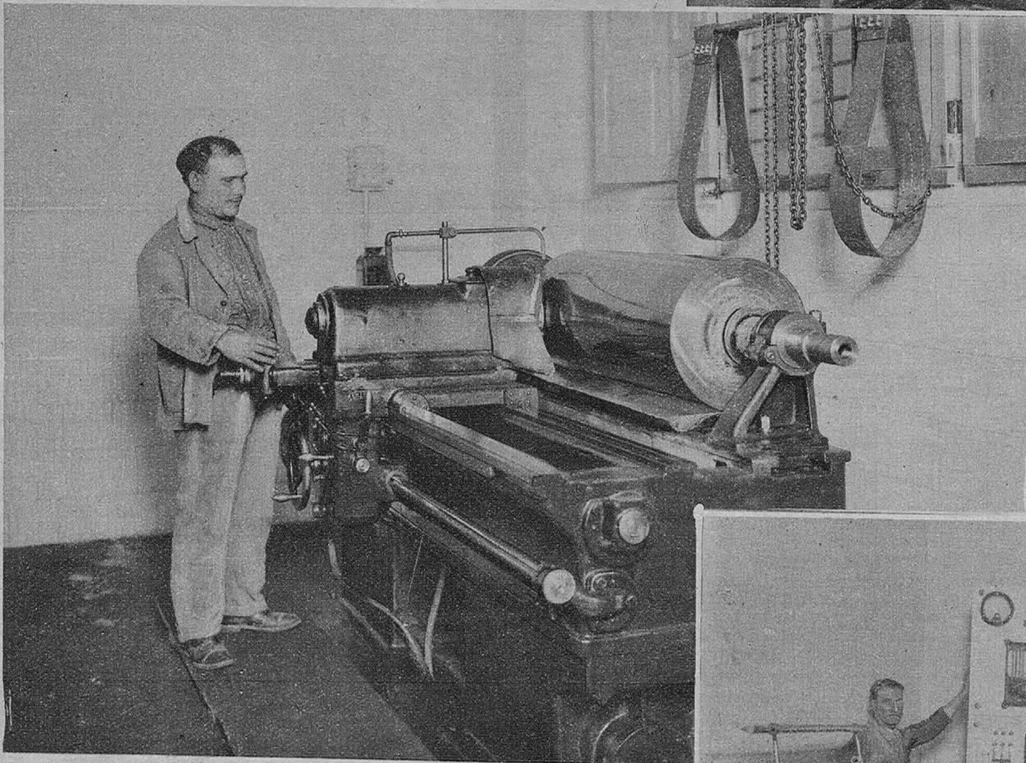
Aparato para borrar los cilindros, después de impreso el periódico.
