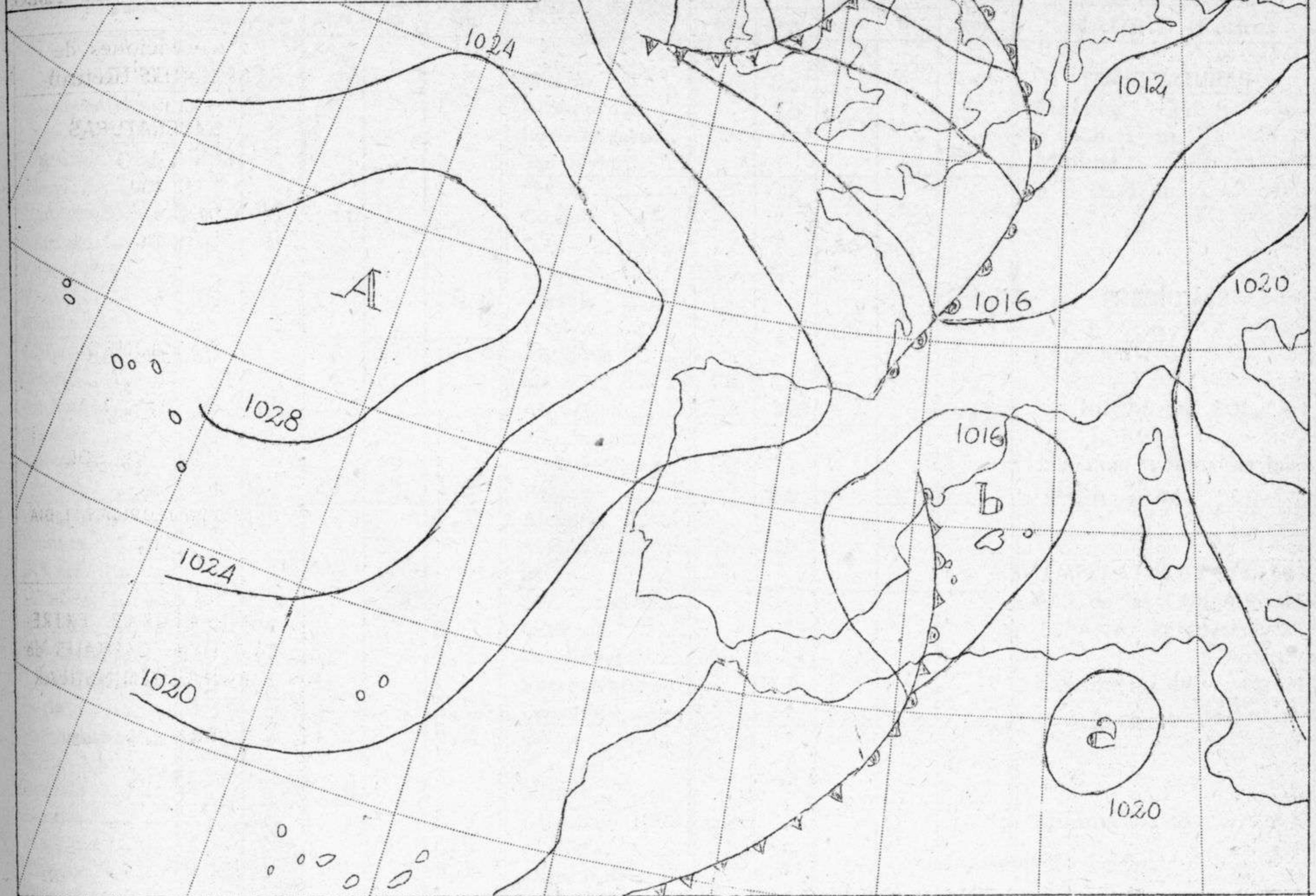
ISOBARAS Y FRENTE a 06 h. T.M.G.
