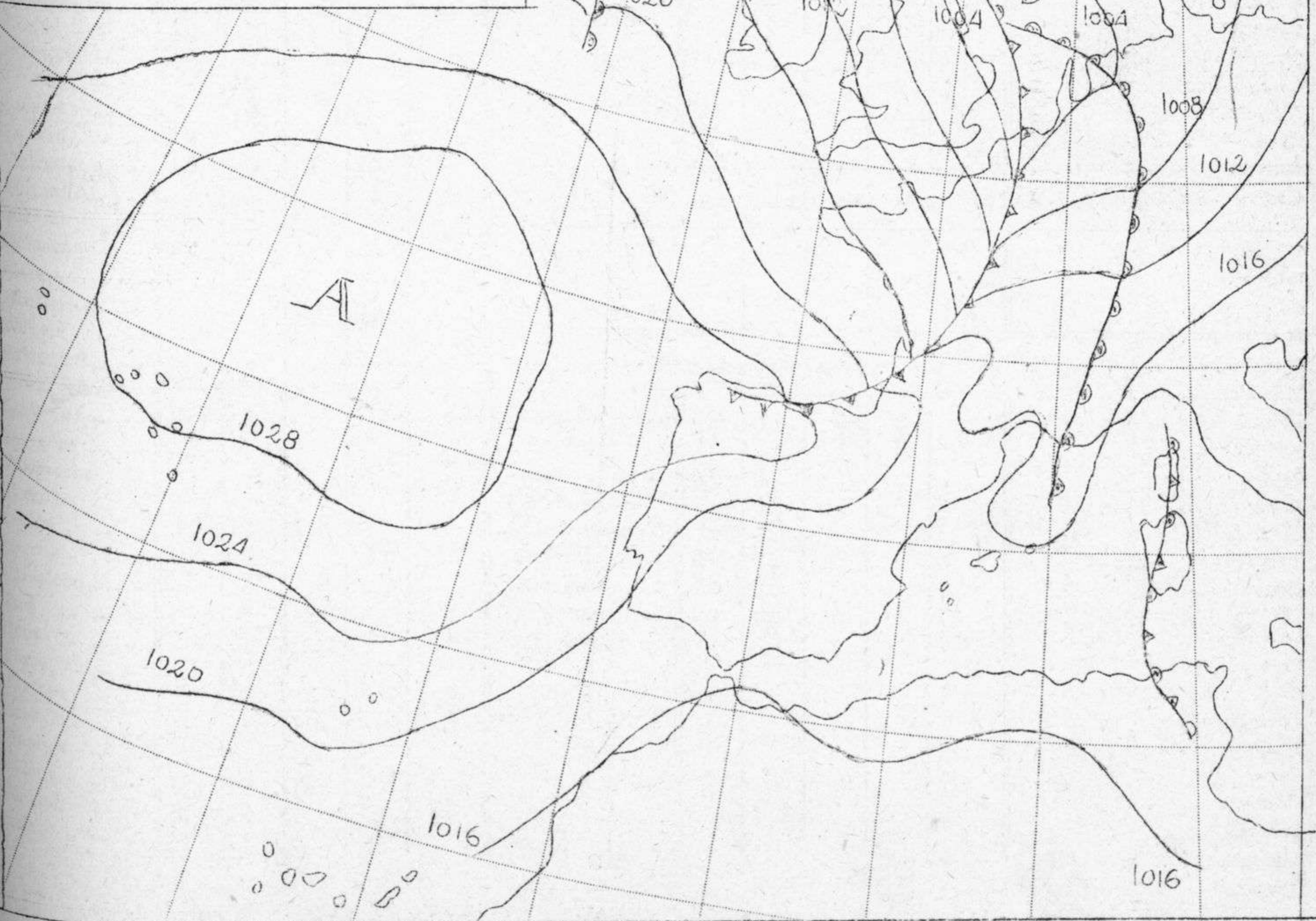
ISOBARAS Y FRENTE a 18 h. T.M.G.
