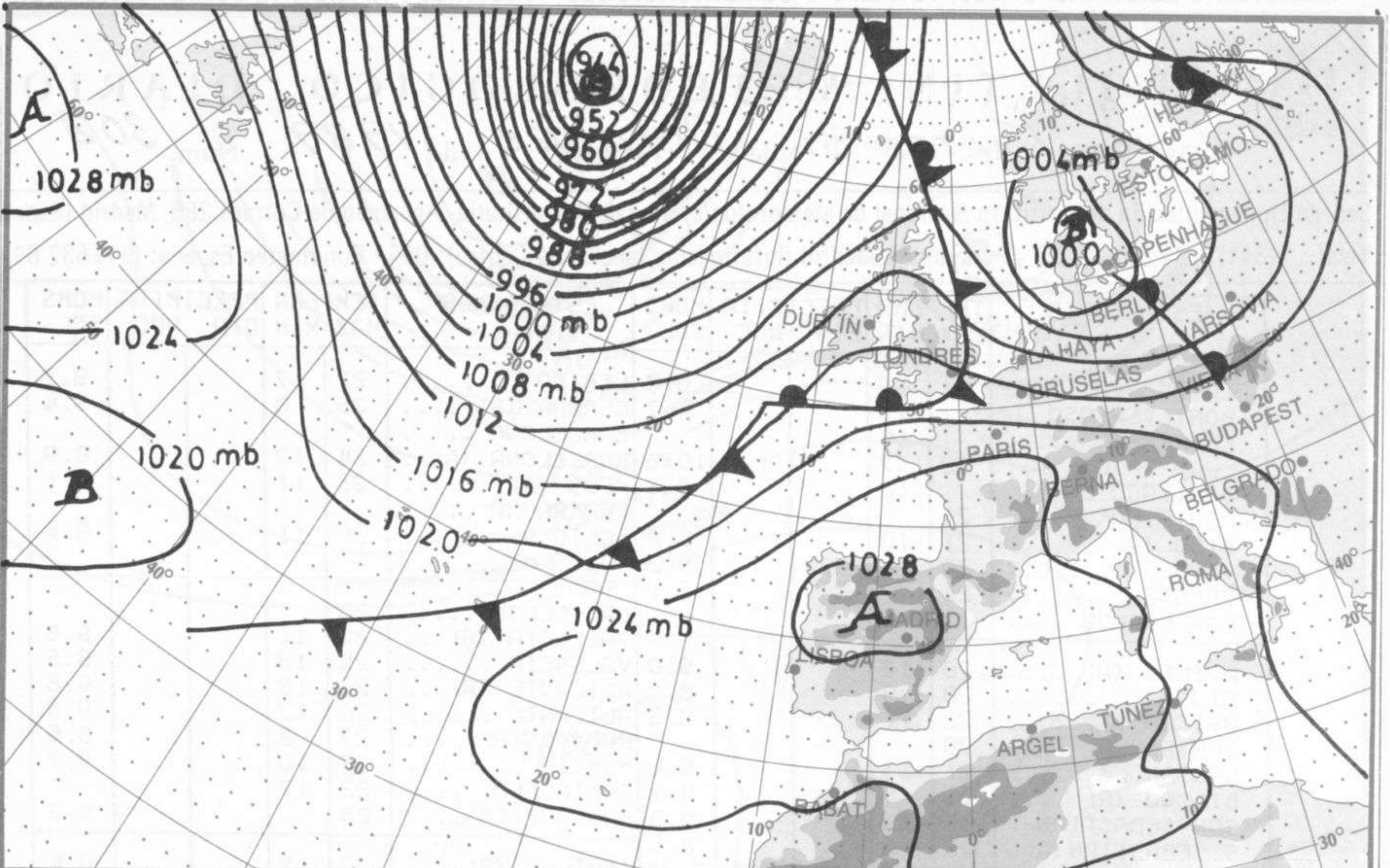
ANALISIS EN SUPERFICIE a 12 h. (TMG) Día 30-10-89
