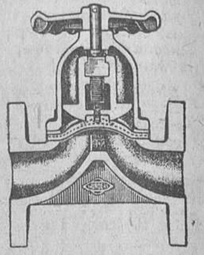
Válvula a diafragma SAUNDERS
