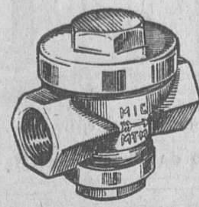
El purgador termodinámico "MIL" para vapor y aire.
