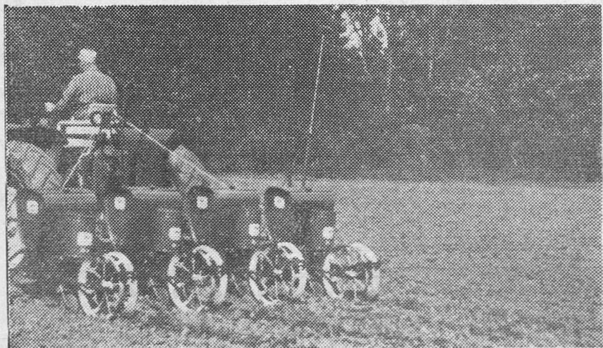
Abonadora sembradora JOHN DEERE localizando el abono en las proximidades de la semilla con el fin de favorecer la nascencia.
