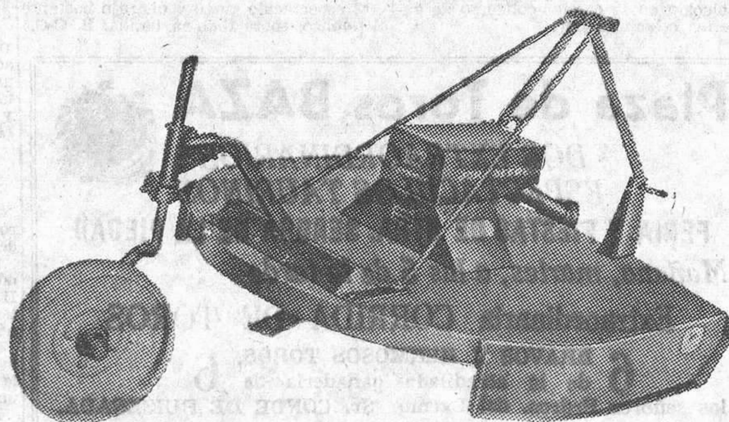
He aquí la máquina desbrozadora "GYRAMOR", creación de John Deere, para hacer más rentable una explotación agrícola. Con ella, en sus modelos 127 y 307, podrá limpiar con poco gasto y escasa mano de obra, los rastrojos del maíz, los residuos del algodón, trocear los sarmientos de la viña, eliminar la maleza que nace entre el arbolado y a lo largo de los edificios, como los viejos pastos, donde abundan las plantas leñosas inútiles para la alimentación del ganado y otras muchas faenas.
