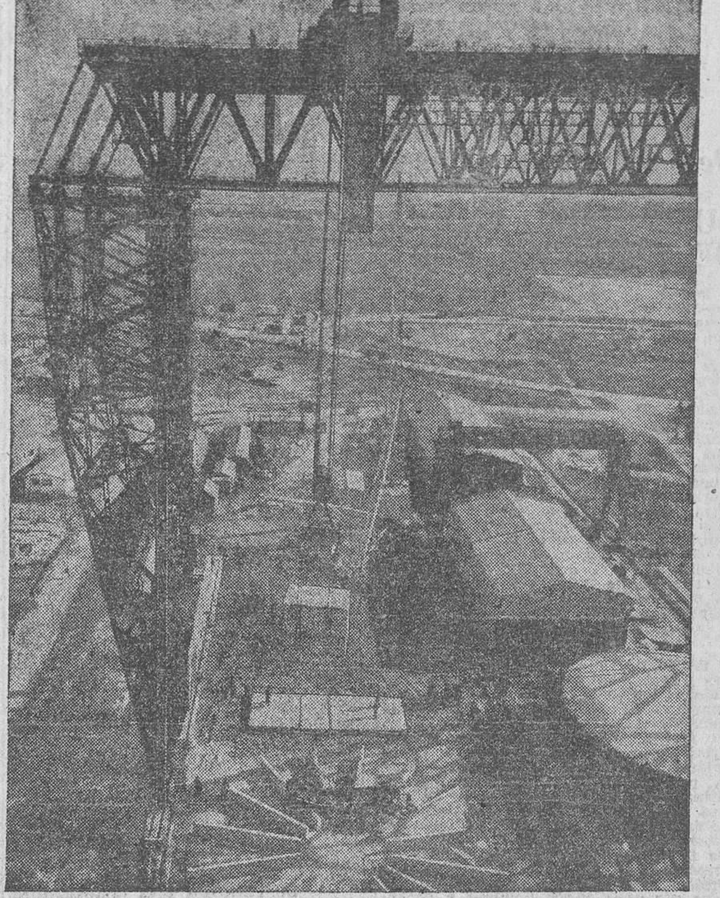
En la construcción de la central electroatómica de Bradwell, Essex (Inglaterra) se ahorra tiempo y dinero con el empleo de esta enorme grúa de 55,5 metros de altura, que es la mayor de su tipo en el mundo. Esta grúa abarca los edificios del reactor y está montada sobre ocho trenes articulados de cuatro ruedas que se deslizan sobre una vía férrea. Este sistema de montaje permite a la grúa transportar calderas pesadas o estructuras del reactor de docenas toneladas de peso a una gran altura sobre el solar de construcción y colocarlas en posición en los reactores sin interrumpir los trabajos en otros edificios.
