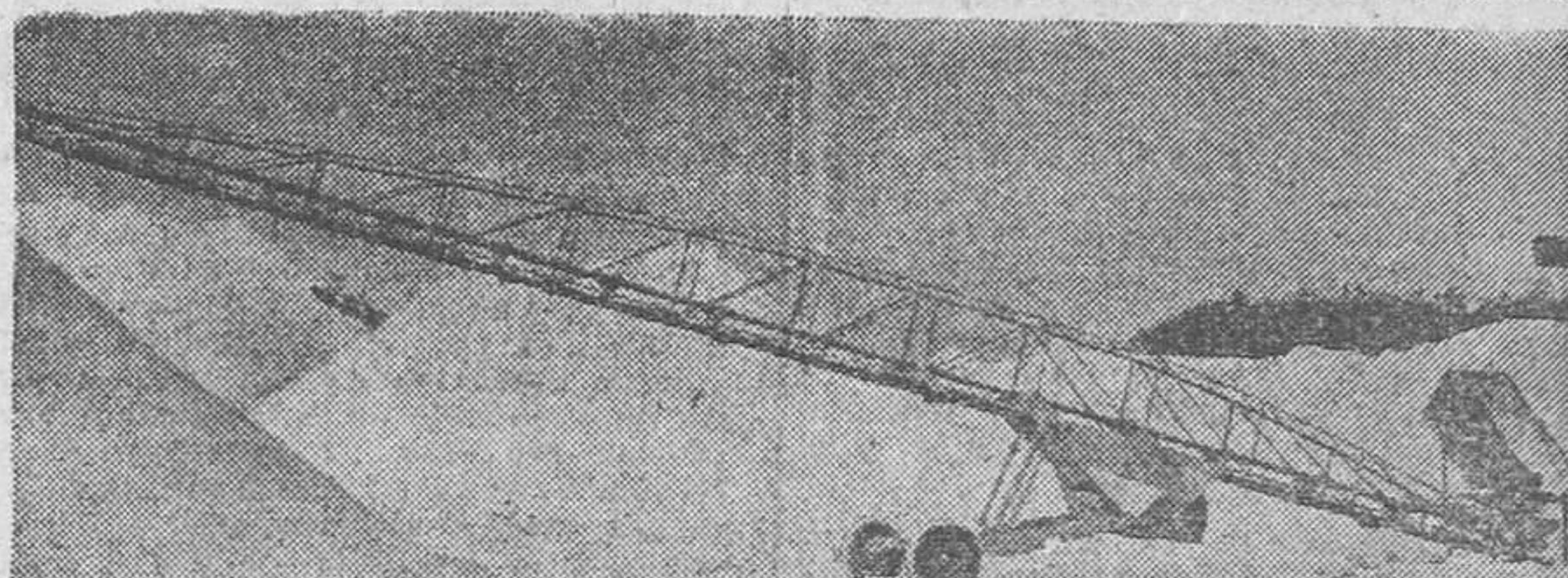
De excelente aseo y con un alto grado de manufactura, esta nueva elevadora británica ha despertado mucho interés, ya que con sus veinte metros de elevación y dos toneladas de peso puede hacer el trabajo para el que normalmente se emplea una máquina de treinta y tantos metros
