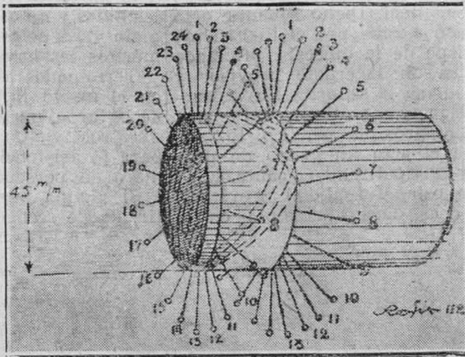
Construcción de las bobinas en forma de abeja. (Figura A.)
