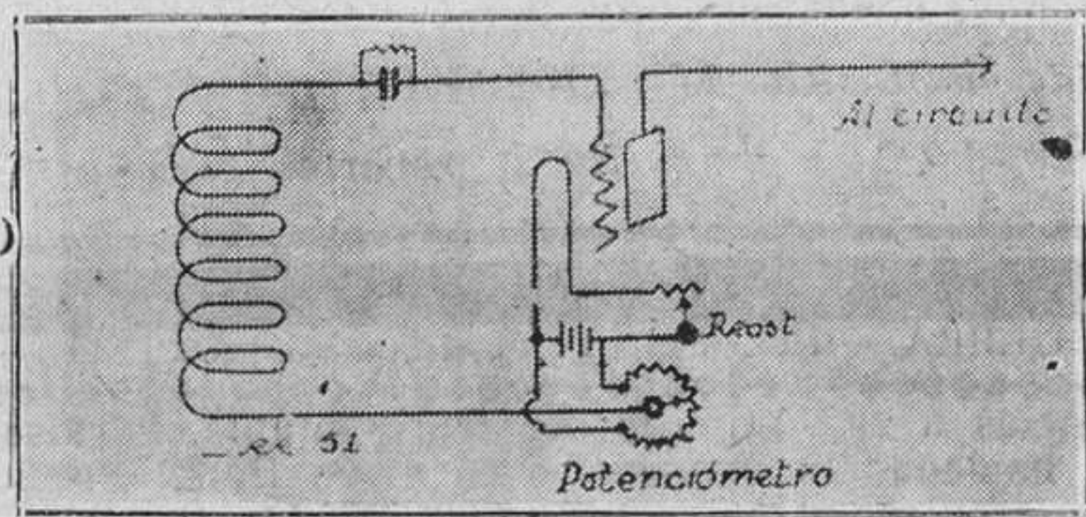
Figura 1.-Colocación de un potenciómetro.
