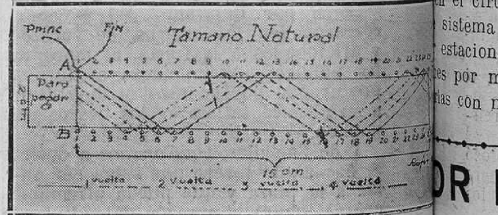
Construcción de las bobinas en forma de abeja. (Figura B.)
